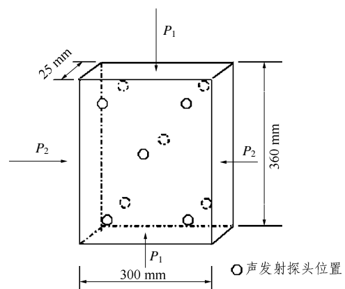
图 2 岩石试样的几何尺寸、声发射探头的分布以及载荷情况
