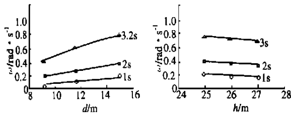
图 5 w 与 d 关系曲线 图 6 w 与 h 关系曲线
