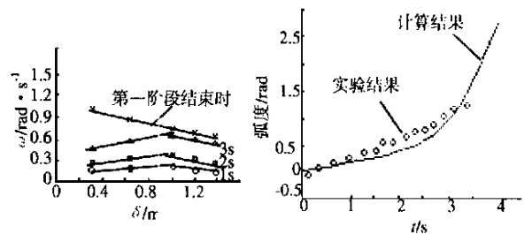
图 7 w 与 \delta 的关系曲线 图 8 计算与实验结果对比
