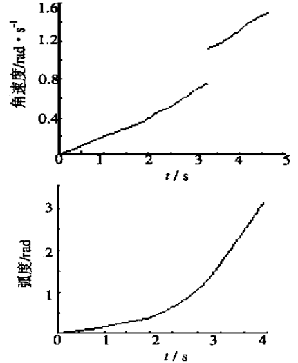
图 4 翻转过程的角度和角速度曲线
