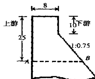
图 1 围堰断面示意图(单位:m)
