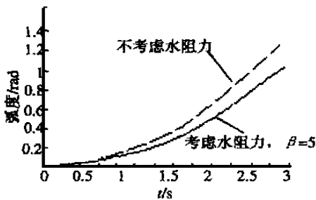
图 10 实际工程尺度下翻转的计算结果
