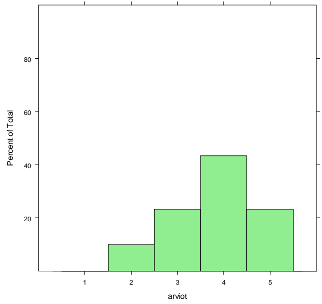
M2_normi_miellyttavyys_S2
