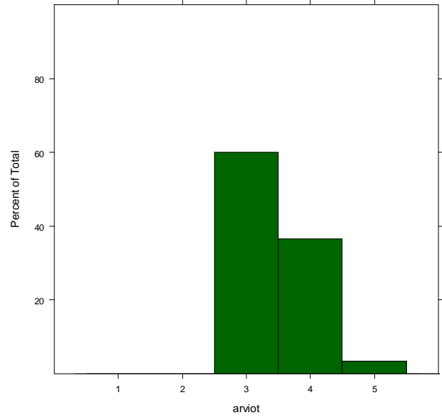
M1_selko_nopeus_S2
