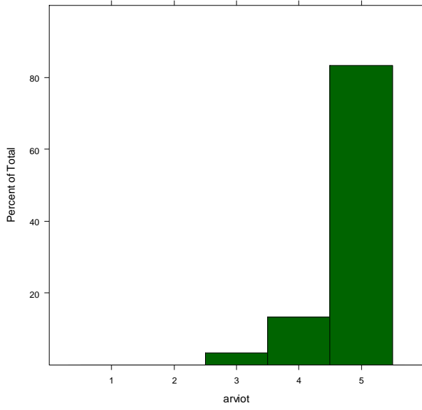
M1_normi_ymmarrettavuys_kontrolli
