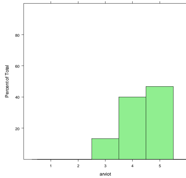
M2_selko_selkeys_S2
