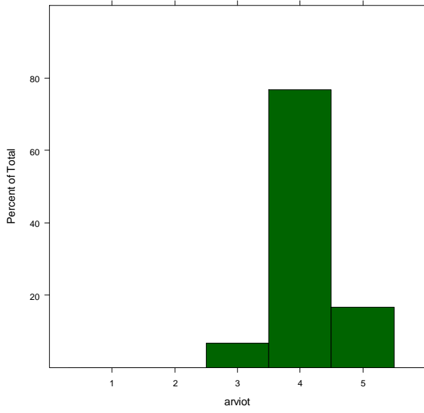
M1_selko_nopeus_kontrolli
