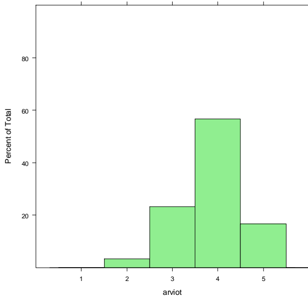
M2_selko_miellyttavyys_kontrolli
