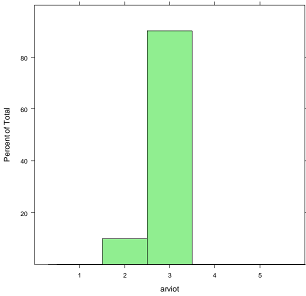
M2_normi_nopeus_kontrolli
