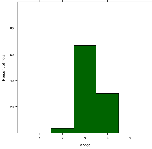
M1_normi_nopeus_kontrolli
