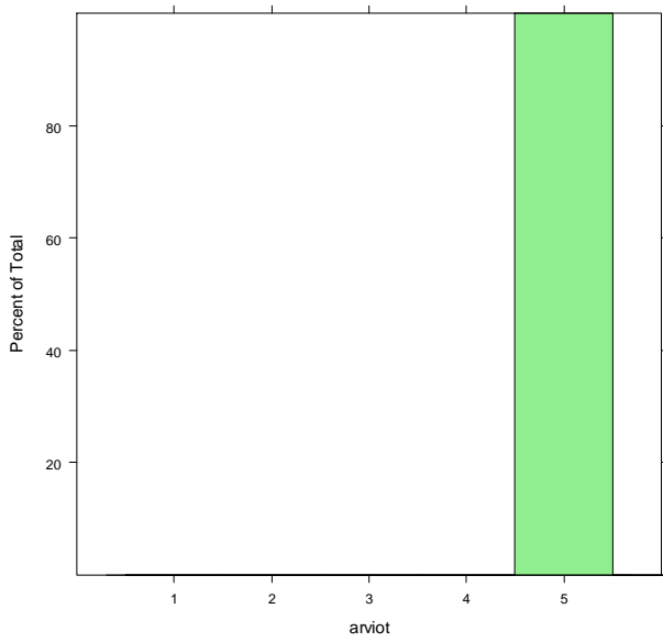
M2_selko_ymmarrettavuys_kontrolli
