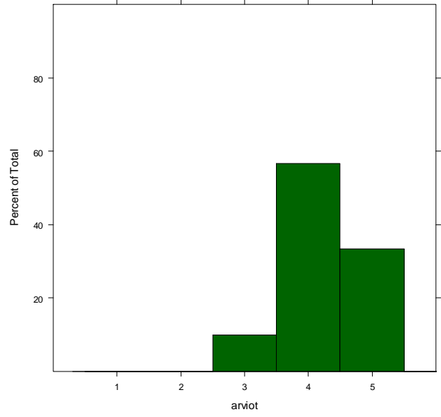
M1_normi_selkeys_S2
