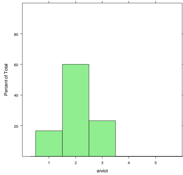
M2_normi_nopeus_S2
