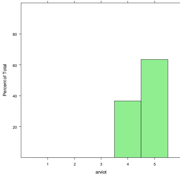
M2_selko_selkeys_kontrolli
