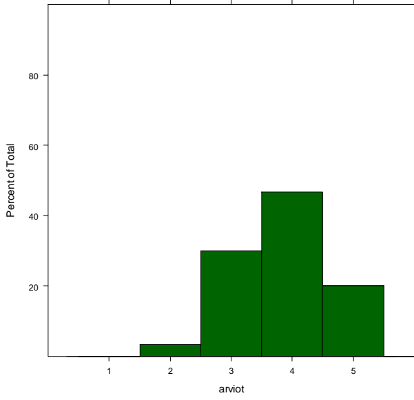
M1_selko_miellyttavyys_kontrolli
