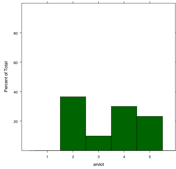
M1_selko_ymmarrettavuys_S2
