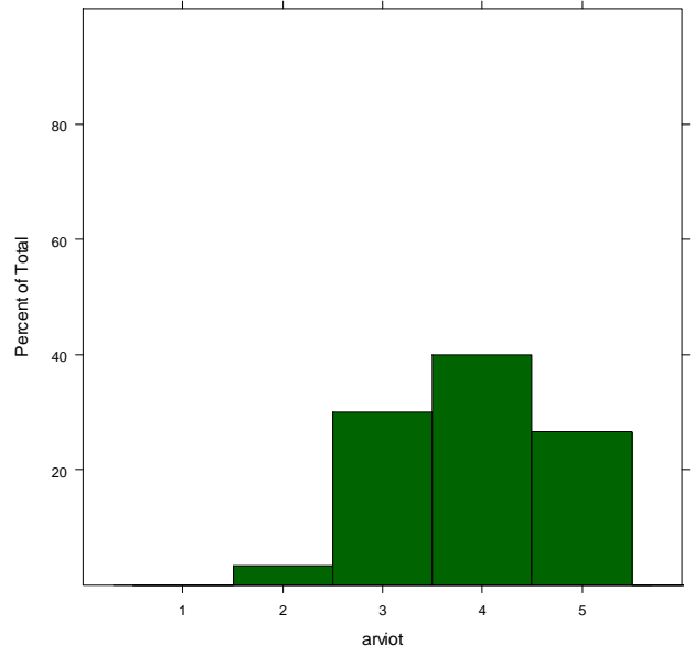
M1_normi_miellyttavyys_S2
