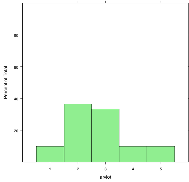
M2_normi_ymmarrettavuys_S2
