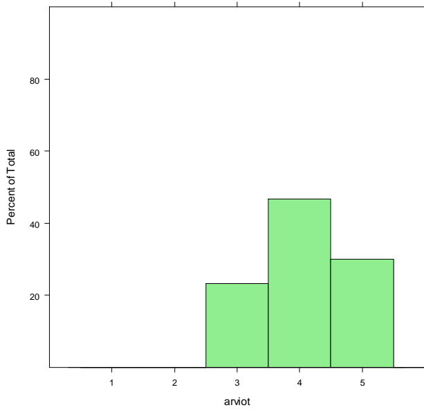
M2_normi_miellyttavyys_kontrolli
