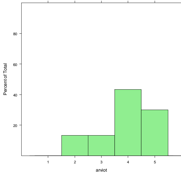
M2_selko_ymmarrettavuys_S2
