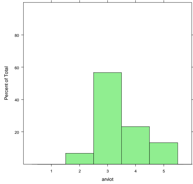
M2_normi_selkeys_S2
