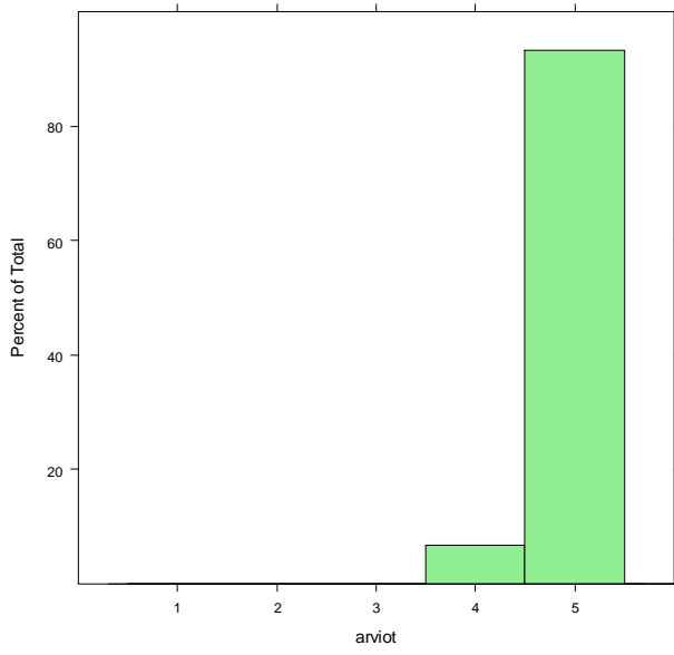
M2_normi_ymmarrettavuys_kontrolli
