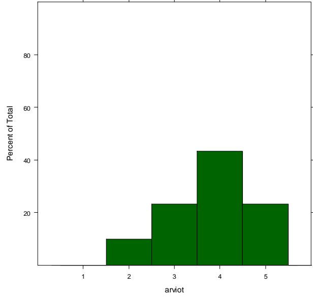
M1_selko_miellyttavyys_S2
