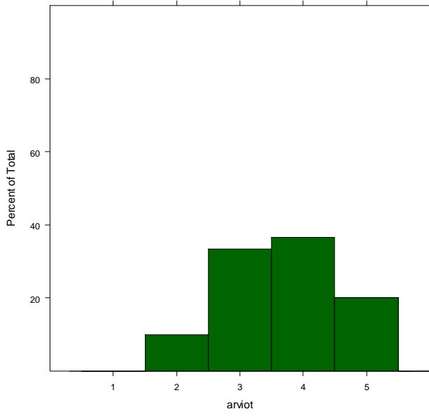
M1_normi_miellyttavyys_kontrolli
