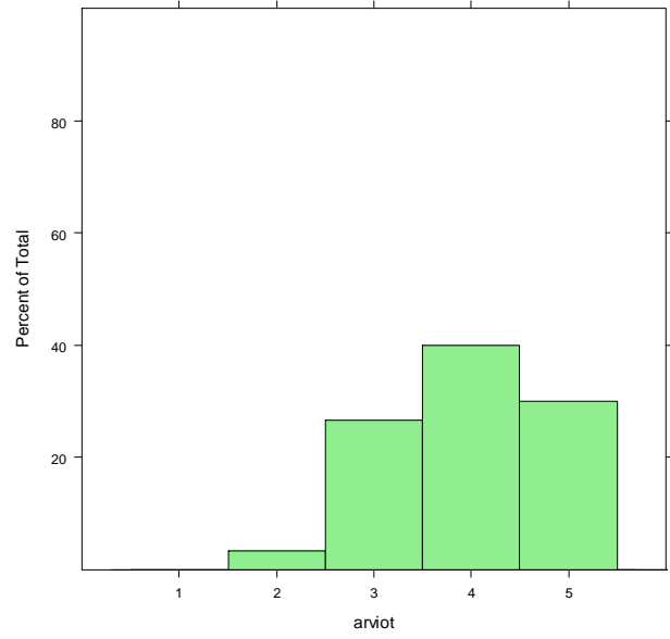
M2_selko_miellyttavyys_S2
