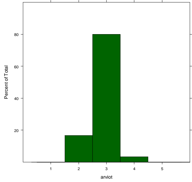
M1_normi_nopeus_S2
