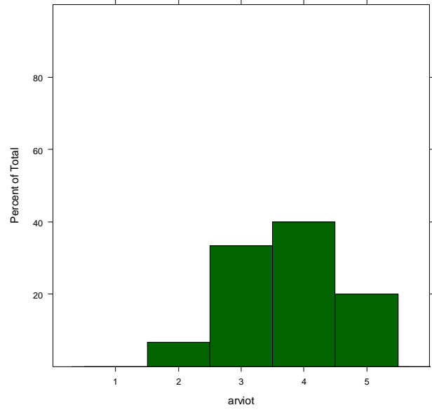
M1_normi_ymmarrettavuys_S2
