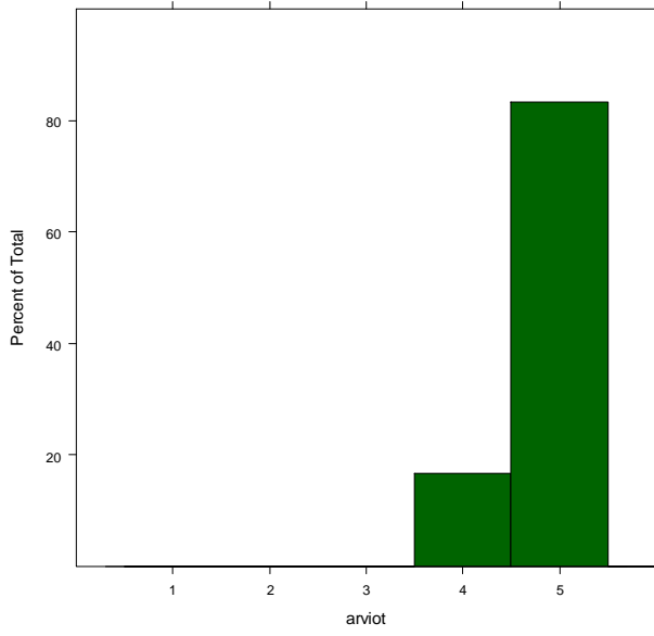
M1_selko_ymmarrettavuys_kontrolli
