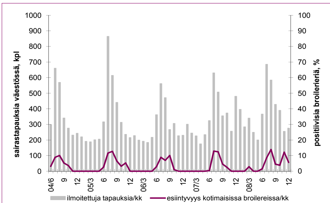
Kuva 2. Kuukausittain ilmoitetut kampylobakterioositapaukset väestössä, sekä kuukausikohtaiset kampylobakteerin esiintyvyydet teurasbroilereilla (Lähde: Valtakunnallinen tartuntatautirekisteri, THL; Kampylobakteerin valvontaohjelma, Evira).
