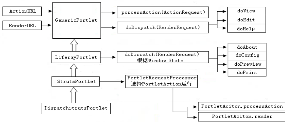
图 3 Portlet 工作流程图
