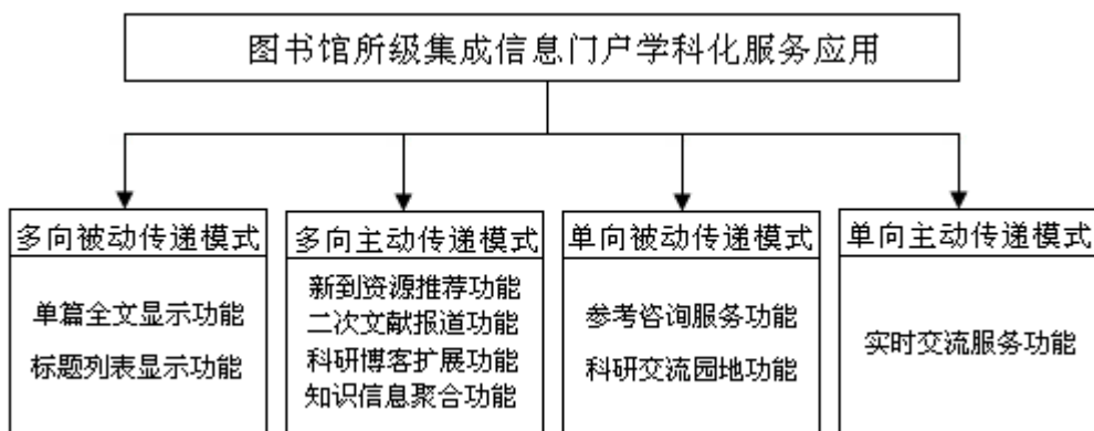
图2 学科化服务信息传递模式整体设计
