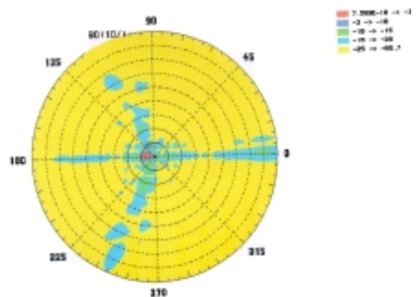
Figura 9. Diagrama de radiación a 12 GHz.
