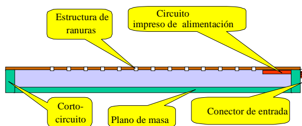
Figura 1. Sección longitudinal de la guía biplaca.
