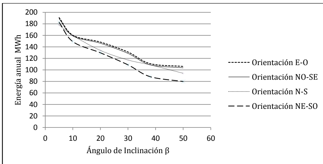
Figura 3. Energía anual en función del ángulo de inclinación del GFV y la orientación del edificio.
