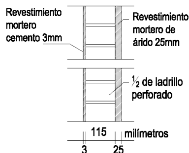
Figura 2 - Muestra de ensayo
