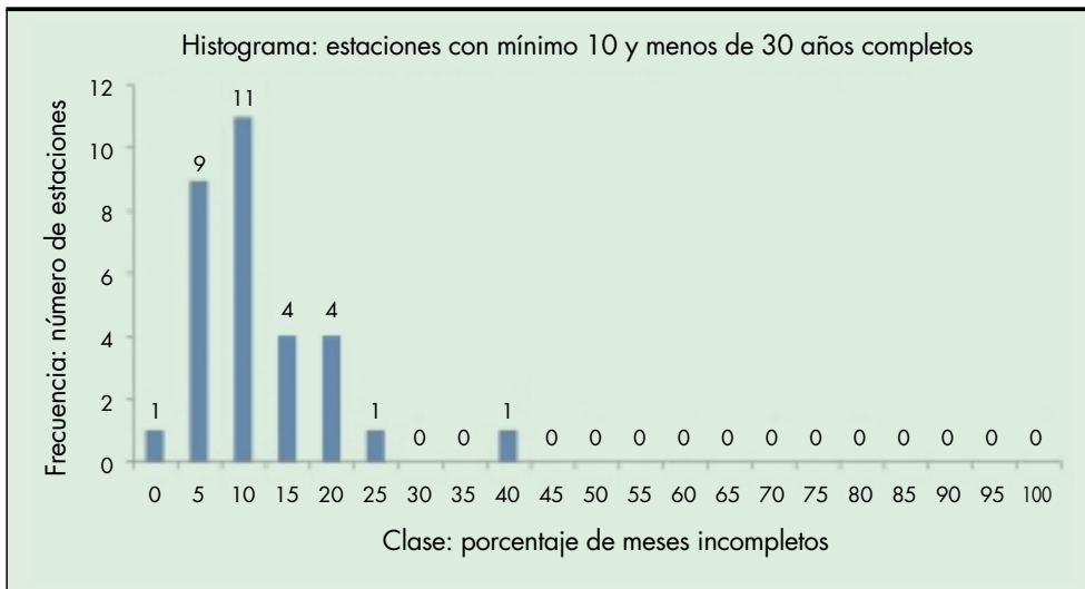
FIGURA 6. Histograma del estudio previo de las estaciones y datos del Guadiana.
