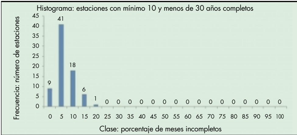
FIGURA 10. Histograma del estudio previo de las estaciones y datos del Ebro.
