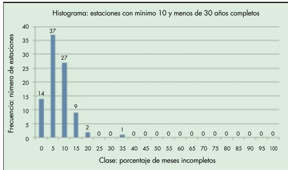
FIGURA 5. Histograma del estudio previo de las estaciones y datos del Tajo.
