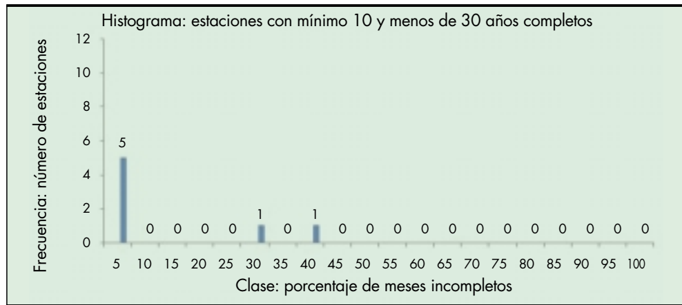
FIGURA 11. Histograma del estudio previo de las estaciones y datos del Miño.
