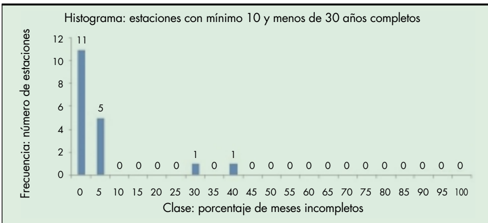
FIGURA 12. Histograma del estudio previo de las estaciones y datos del Cantábrico.
