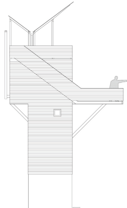
Figura 10. Reconstrucción gráfica de la cabaña de Oropesa de F. J. Sáenz de Oíza. Alzado este.
