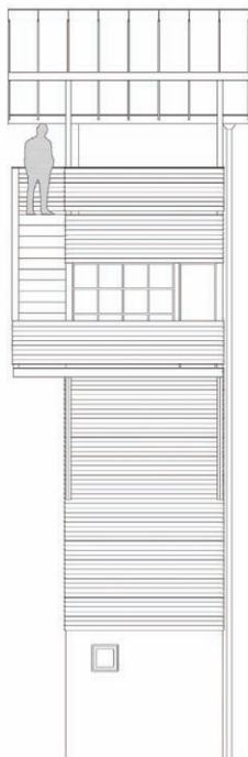
Figura 9. Reconstrucción gráfica de la cabaña de Oropesa de F. J. Sáenz de Oíza. Alzado norte.
