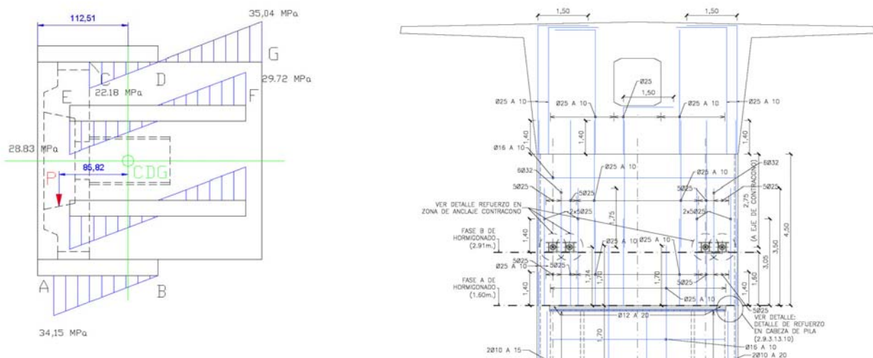
Figura 16. Obtención de tensiones y localización de refuerzos (ULMA e IDEAM-FHECOR)
