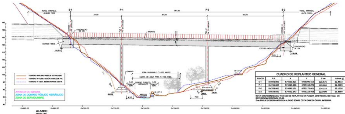
Figura 1. Alzado correspondiente al Viaducto sobre el Arroyo Salubita.
