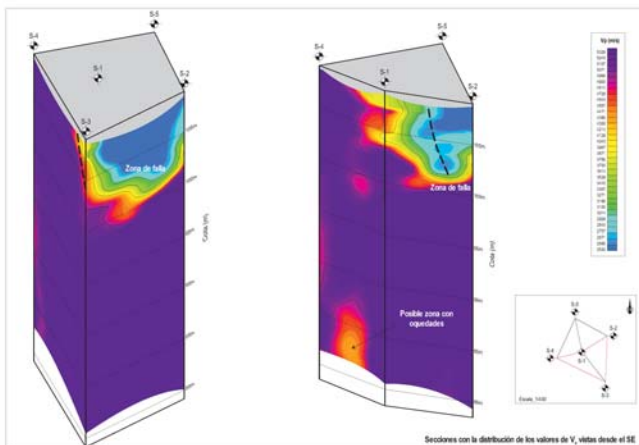
Figura 18. Levantamiento geofísico para del terreno de cimentación
