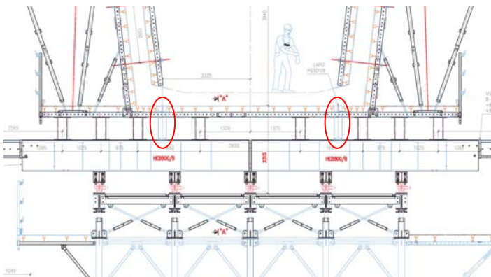
Figura 12. Ubicación de los “lápices”
