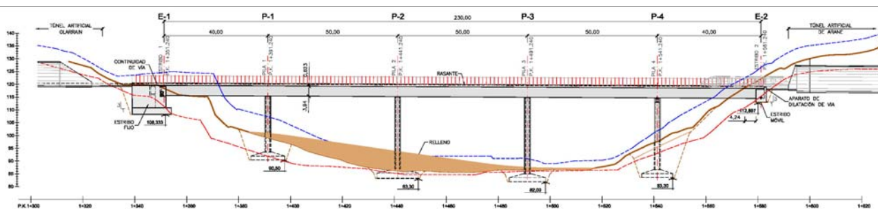
Figura 2. Alzado correspondiente al Viaducto sobre la Cantera de San Esteban.
