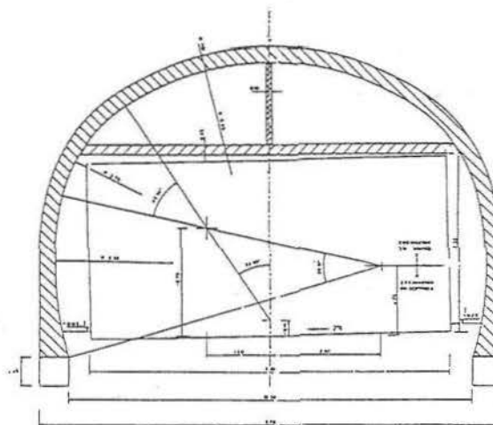
Figura 2.1. Sección transversal del túnel de Somport.
