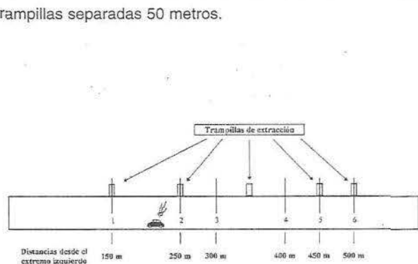
Figura 3.5. Localización de secciones en el túnel
