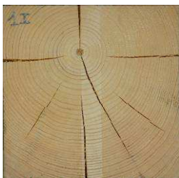
Figura 5. Testa más desfavorable de la pieza 1.
