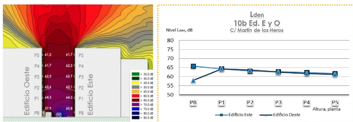
Figura 2– 10b. C/Martin de los Heros. Comparación de Niveles en fachadas y la influencia del aparcamiento.
