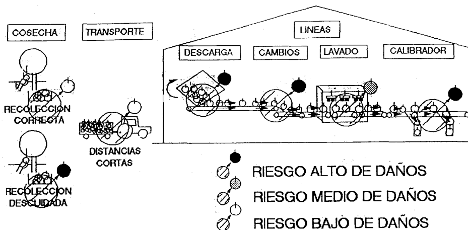
Figura 1: Riesgo de aparición de daños por magulladura en diversas operaciones de manipulación de fruta, según los registros obtenidos por los frutos electrónicos SEP-1 e IS-100.
