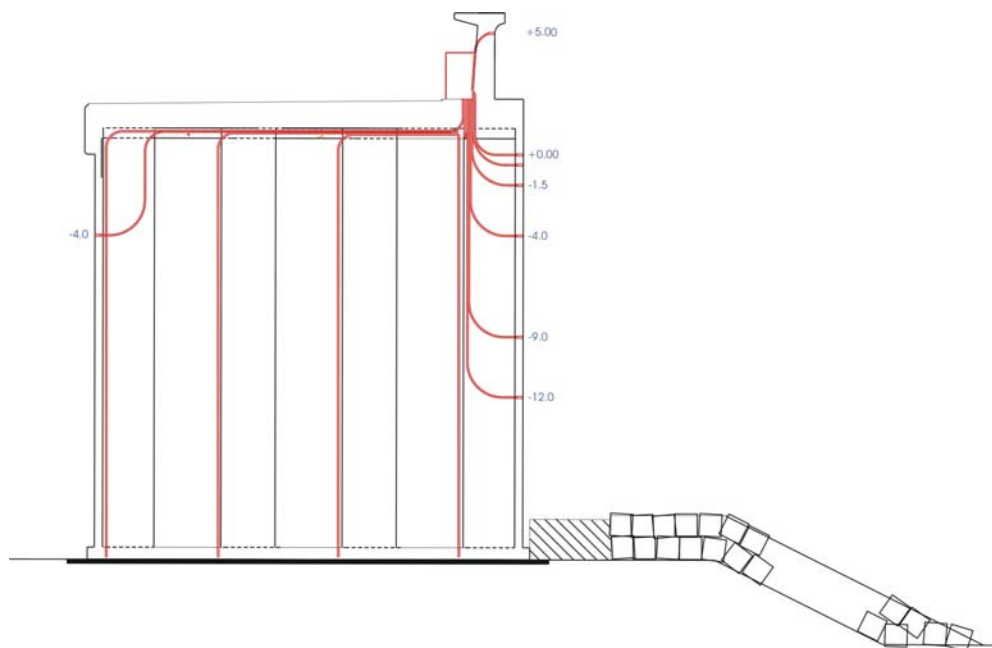
Figura 2. Sección instrumentada con doce sensores de presión y subpresión.
