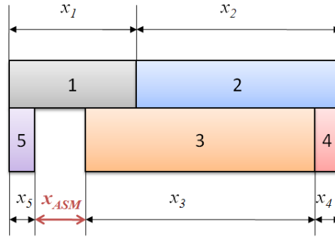
Figura 2. Esquema de ensamblaje (restricción geométrica única)
