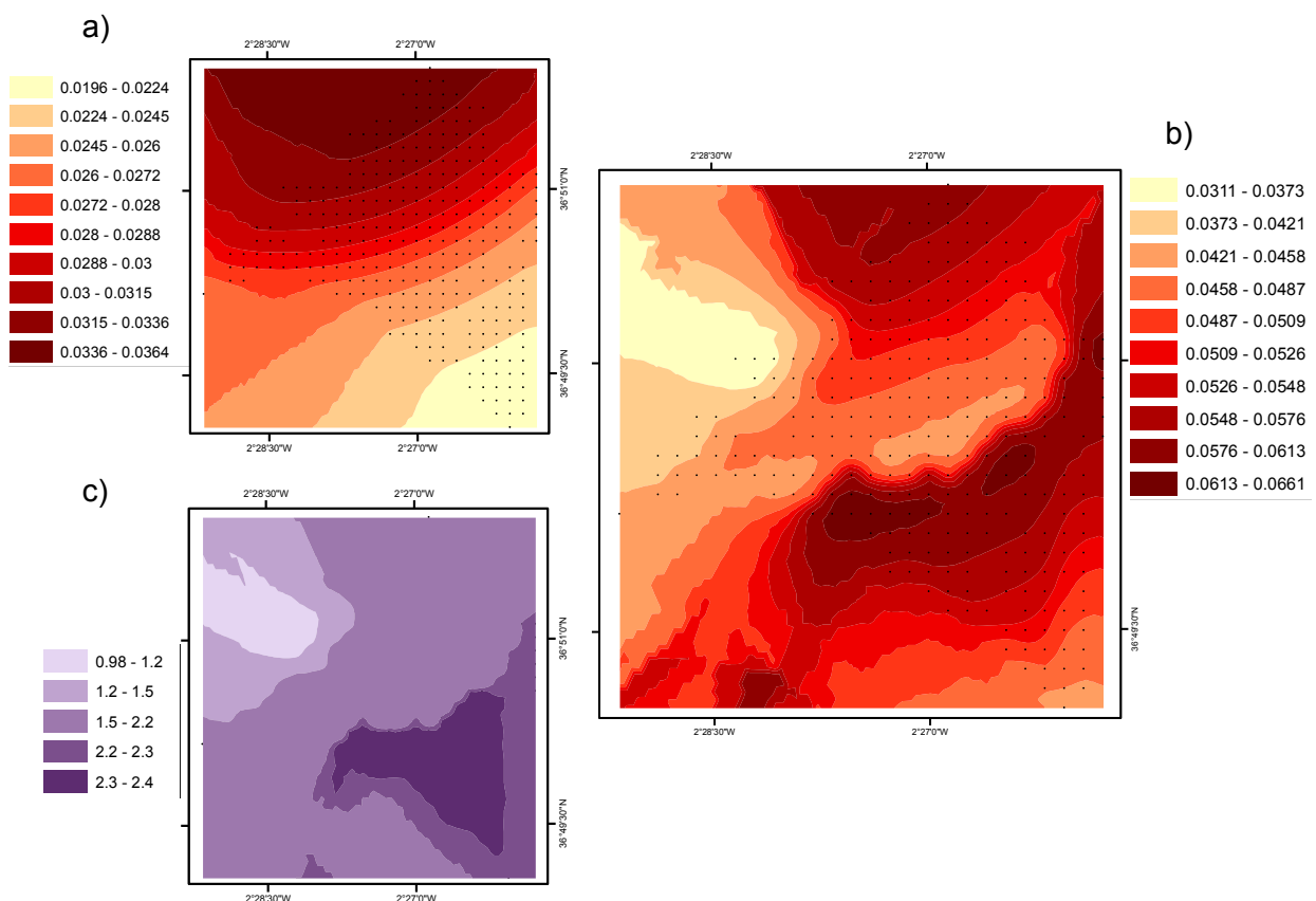
Figura 4. Resultados para el escenario 1 de Almería. a) Mapa de SA(1s) esperada en roca; b) factores de amplificación predichos; c) Mapa de SA(1s) esperada incluyendo efectos de sitio.
