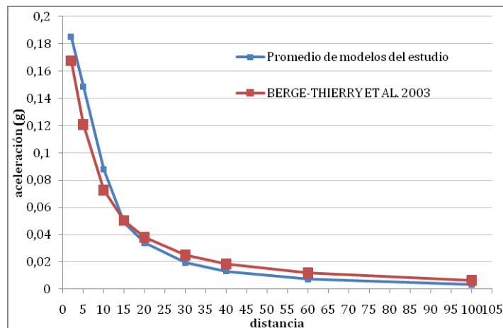
Figura 3. Curvas de atenuación de la PGA con la distancia para un terremoto de magnitud 6.
