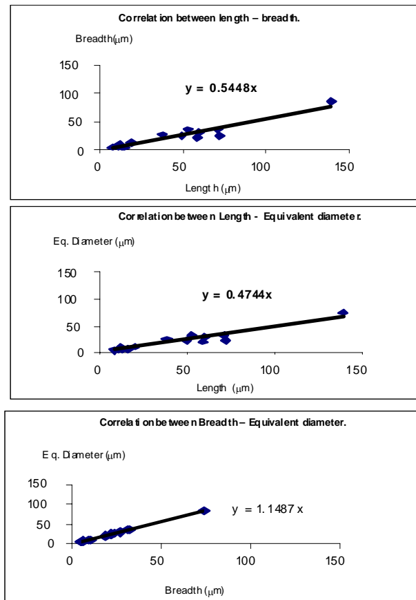
Figura 7. Correlación entre parámetros geométricos obtenidos de los granos de Au en Vetas Guesa y Bruja.
