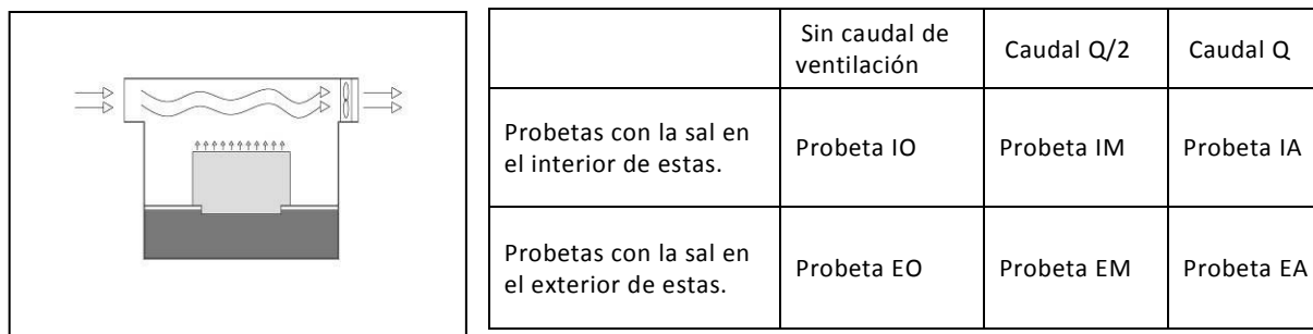
Figura 1.- Diagrama de los contenedores.
