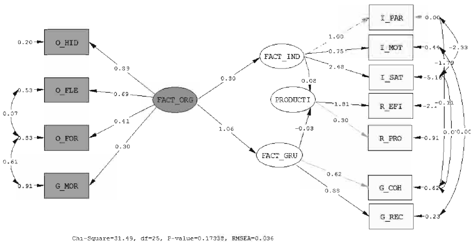
Figura 9 Solución estandarizada del Modelo B, arrojada por LISREL8.80
