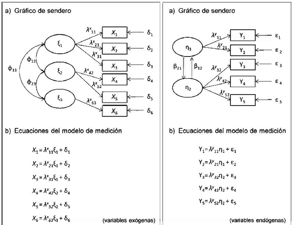
Figura 3 Modelo de medición
