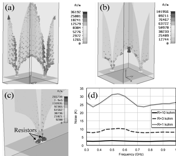
Fig. 3. Corrientes diferenciales a 500 MHz (a); corrientes en modo común a la frecuencia de la anomalía (b); solución propuesta para disipar las corrientes en modo común (c); e incremento extra de ruido debido a las resistencias (d).
