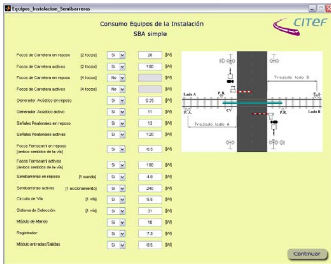
Figura 5 Potencias consumidas.
