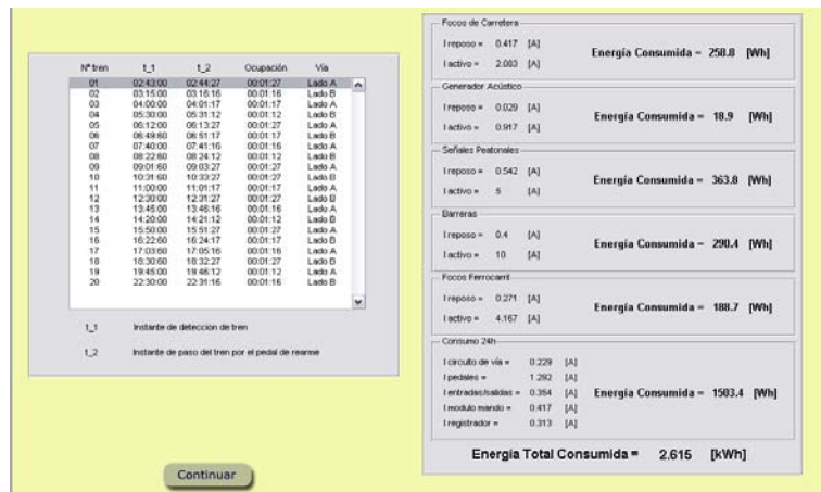
Figura 7. Cálculo de la energía teórica consumida.
