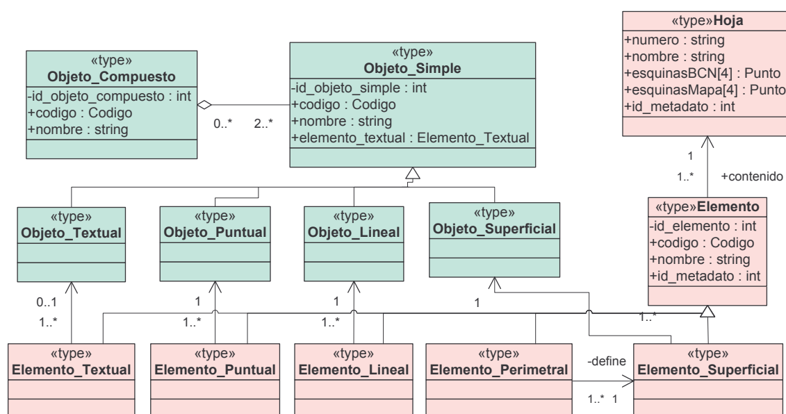
Figura 3. Modelo de clases UML que refleja la división en hojas Modelo de datos v.1.6. Instituto Geográfico Nacional
