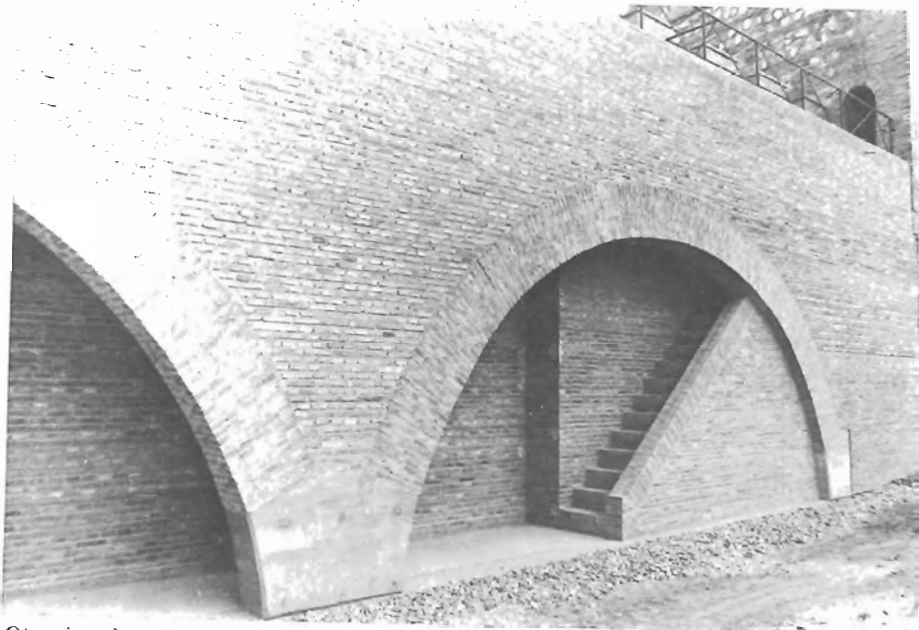
Otro ejemplo reciente de analogía no mimética. Consolidación y reconstrucción de las murallas de Alcalá de Henares. Obra de la Dirección General de Bellas Artes. (Arquitectos: J. Alonso-Martínez y R. Engel).
