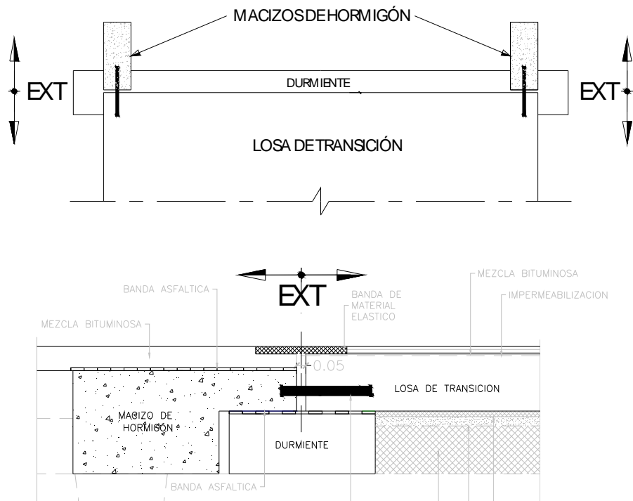
Fig.4a Medición de los movimientos del puente. Disposición de medidores de abertura de junta, al final de las losas de transición.
