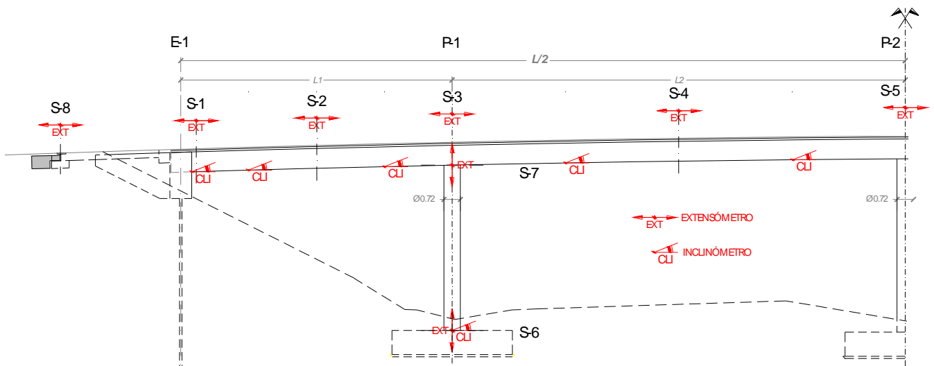
Fig. 2 Esquema de instrumentación. Vista Lateral de la mitad instrumentada del puente.
