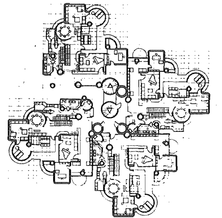
Torres Blancas, de Sáenz de Oiza: planta corbuseriana , planta wrightiana y planta final; vista y esquemas del borde de terrazas y volúmenes.
