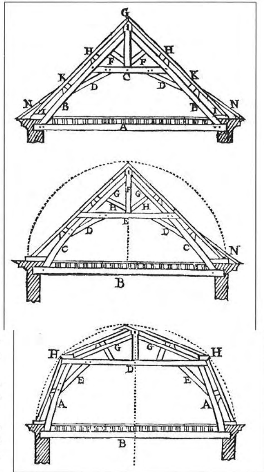
Figura 11 Armaduras de cubierta descritas por Bullet.
