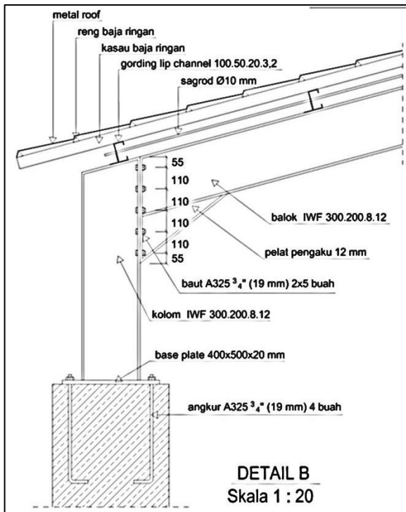
Gambar 2. Detail sambungan kuda-kuda IWF
