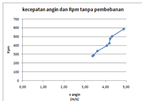
Gambar 14. Grafik kec. angin dan Rpm
