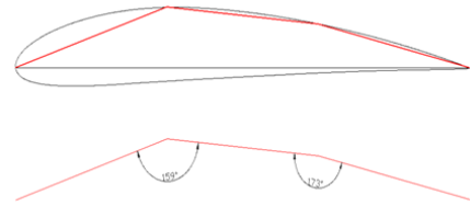
Gambar 2. Profil NACA 4412
