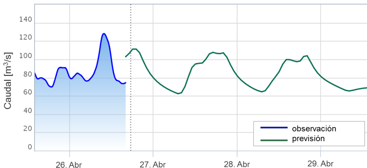
Figura 5.- Desfase entre el caudal observado y el simulado al inicio de la previsión hidrológica (© CREALP, 2016).
