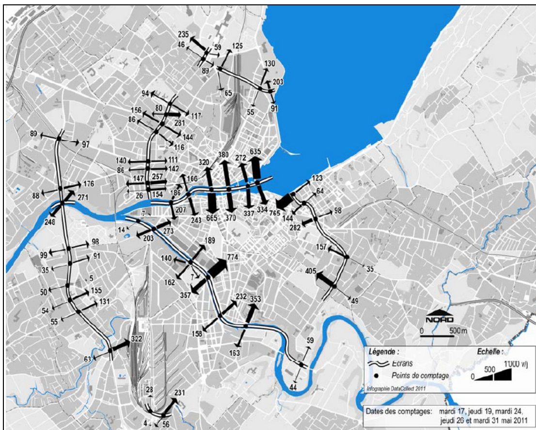
Figure 81: Trafic journalier vélo, juin 2011 source comptages DGM
