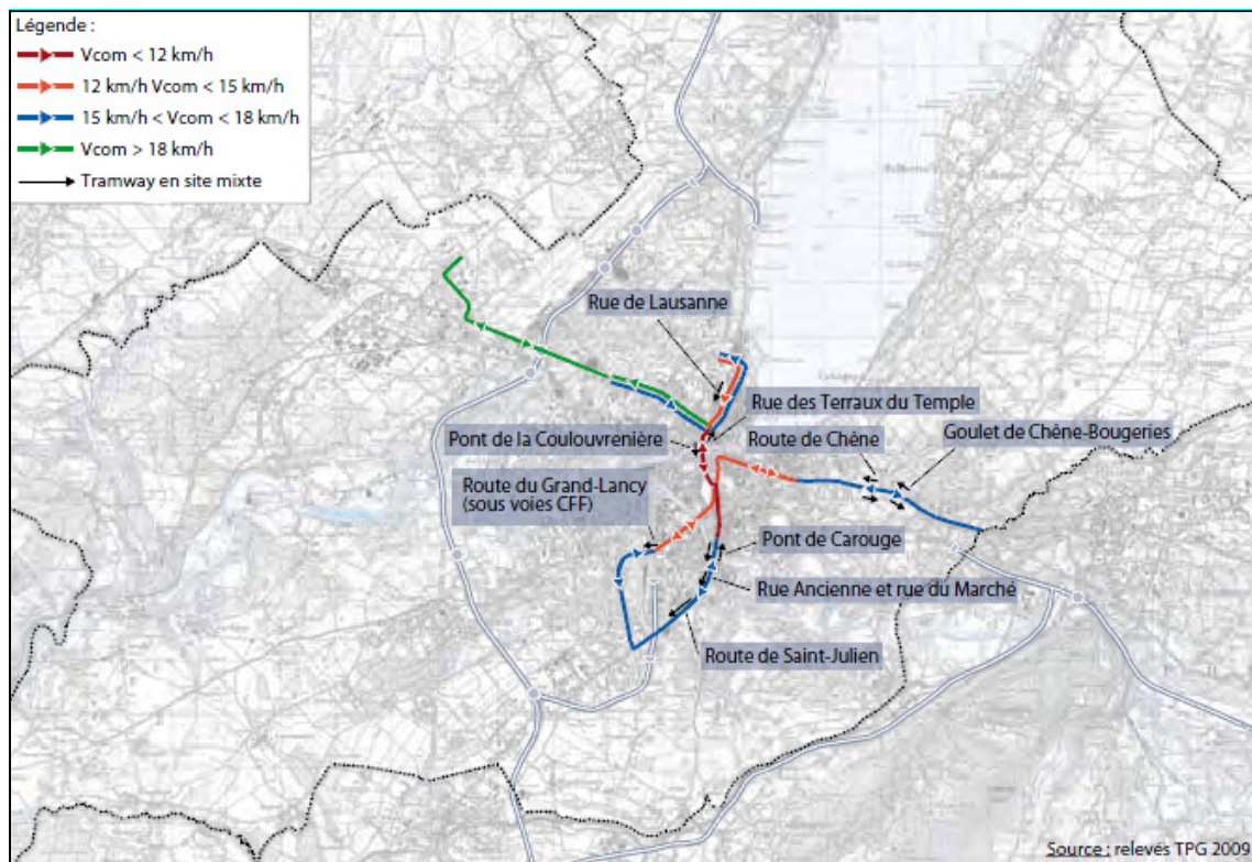
Figure 65: Vitesses commerciales des tramways (progression diurne) source : relevés TPG 2009/PDRR
