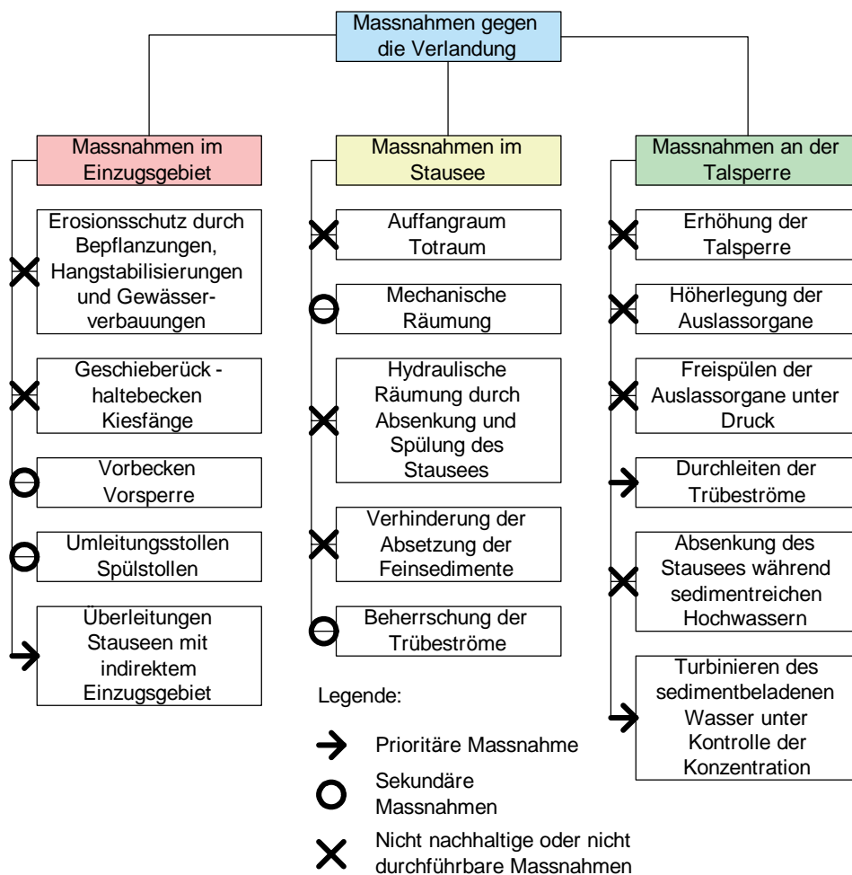
Abb. 6: Übersicht über denkbare Massnahmen gegen die Verlandung (Schleiss, 2005), unterteilt in prioritäre, sekundäre und nicht nachhaltige/nicht durchführbare Massnahmen für die Anlagen der KSL.
