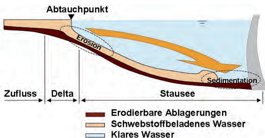
Abb. 3: Schematische Darstellung des Sedimenttransports durch Trübestrome in Stauseen (Oehy und Schleiss, 2003).
