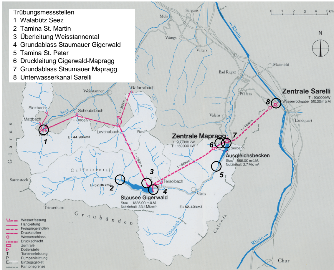
Abb. 1: Übersicht der Kraftwerksanlagen Sarganserland mit den installierten Trübungsmesssonden.
