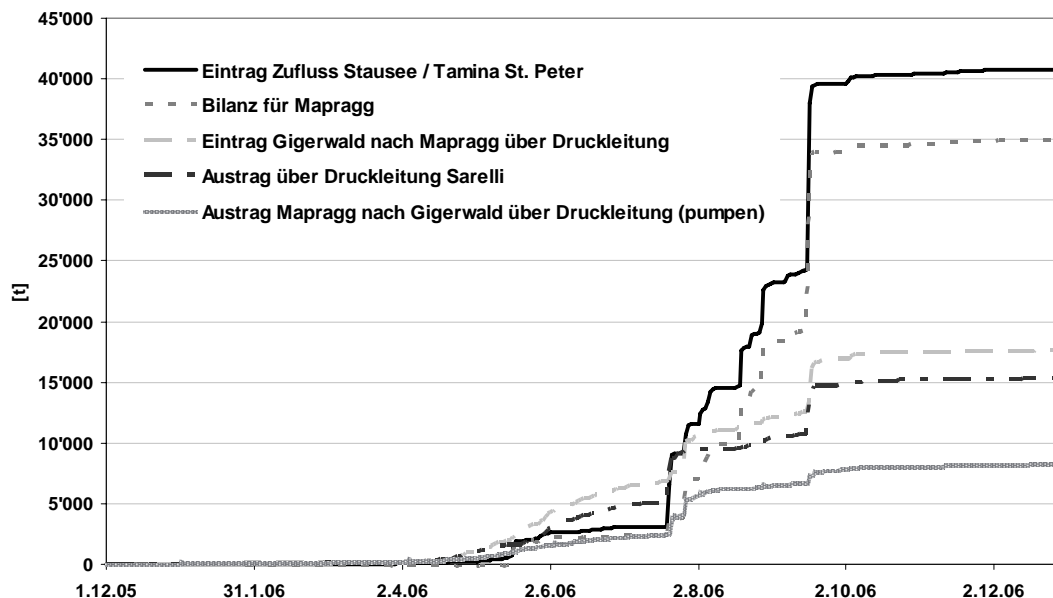
Abb. 5: Summenkurven der Feststofffrachten Mapragg für 2006 (Eintrag und Austrag).
