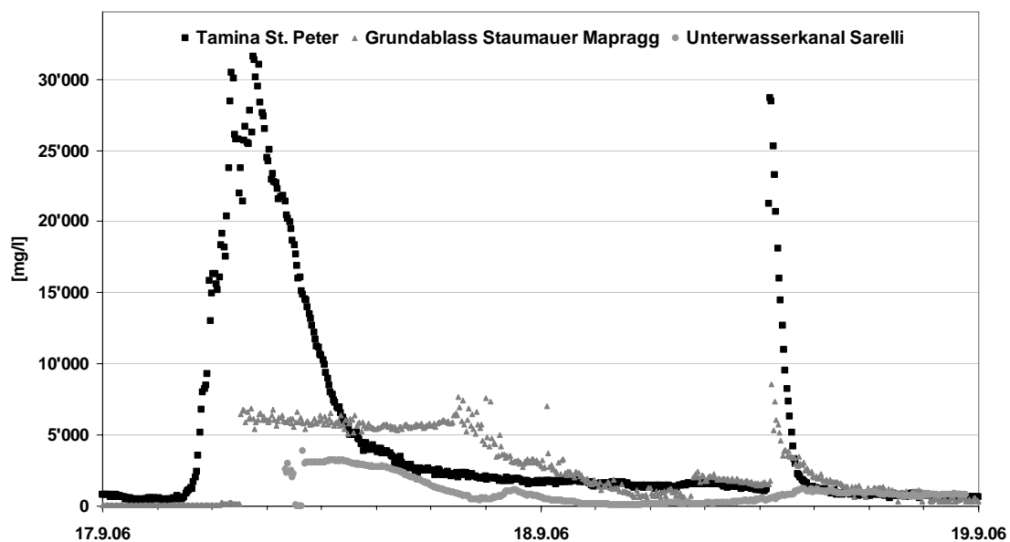
Abb. 4: Messungen der Feststoffkonzentration in Mapragg während den Hochwasser vom 17. und 18. September 2006.
