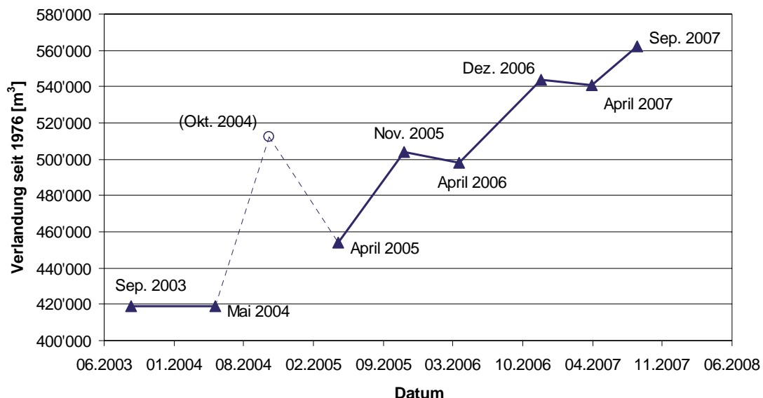
Abb. 2: Verlandungsvolumen Stausee Mapragg gegenüber dem Ausgangszustand von 1976 (Messwert von 2004 vermutlich Fehlmessung).
