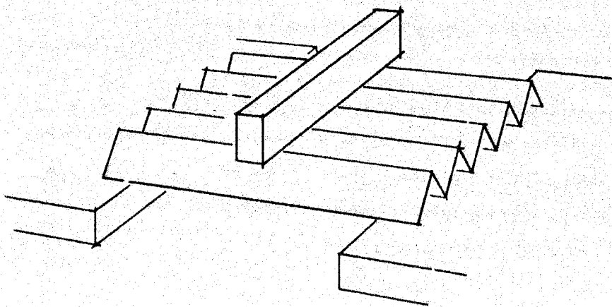
Akkordeonfaltung: Das statische Prinzip der Falte nach Siegel.
