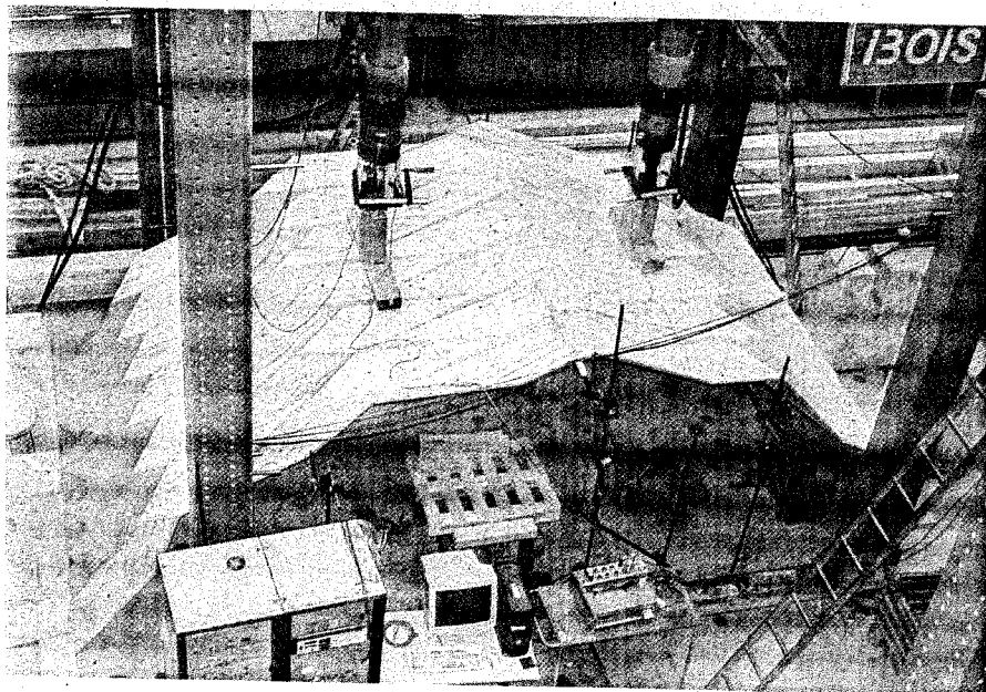
Prototyp: Belastungsversuch.
