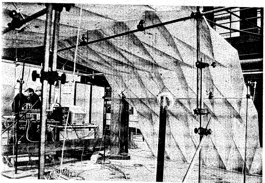
Prototyp der Versuchsanordnung.
