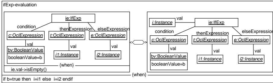
Fig. 21 If-Expression Evaluation
