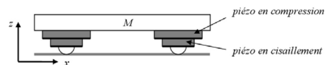
Schéma du chariot pieds vibrants
