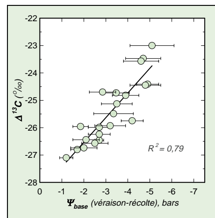
Fig. 2. Relation établie entre le rapport isotopique du carbone ( \Delta^{13}C ) dans les sucres des moûts à la vendange et les valeurs de \Psi_{base} , mesuré durant la période de la maturation à la récolte sur un réseau de 21 parcelles. Barres horizontales: erreur standard. Chasselas, canton de Vaud (CH), 2003.
