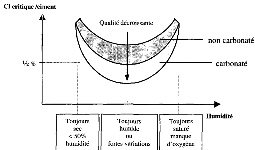
Figure 3.26 Influence de l'enrobage et de l'environnement sur la teneur en chlorures critiques [BREIT_97]
