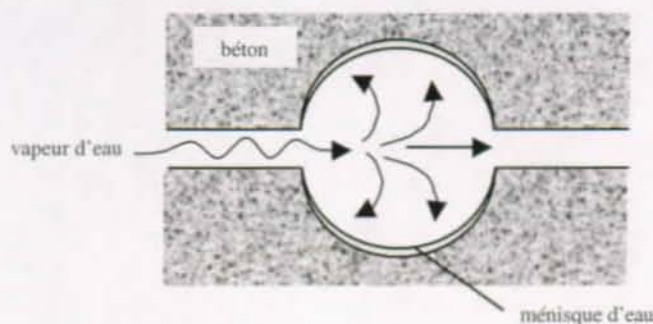
Figure 3.5 Formation de ménisques dans le béton très sec sur la surface des pores.
