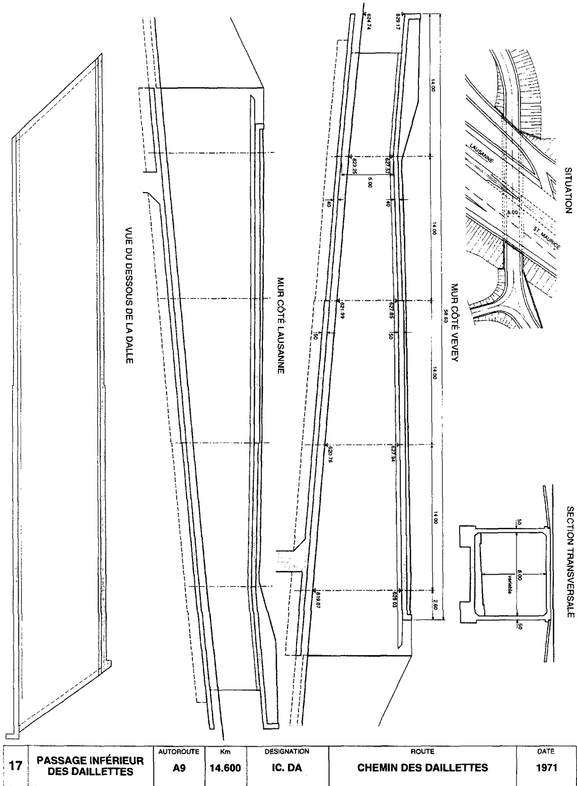
Figure A.7 Plans du pont N°17.
