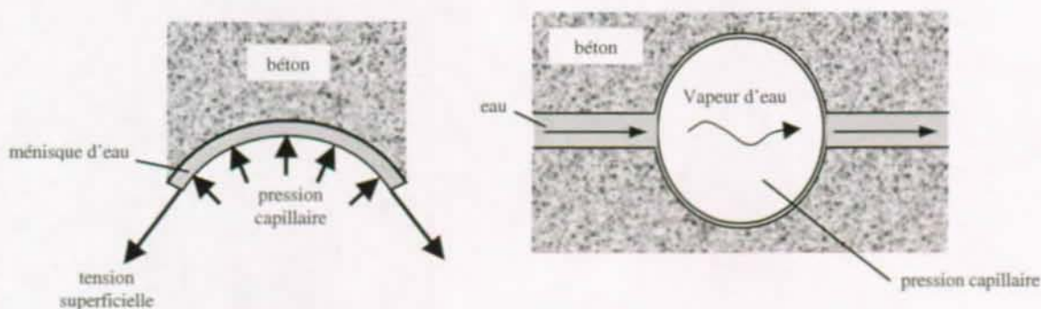
Figure 3.6 Equilibre et condensation capillaire de l'eau.
