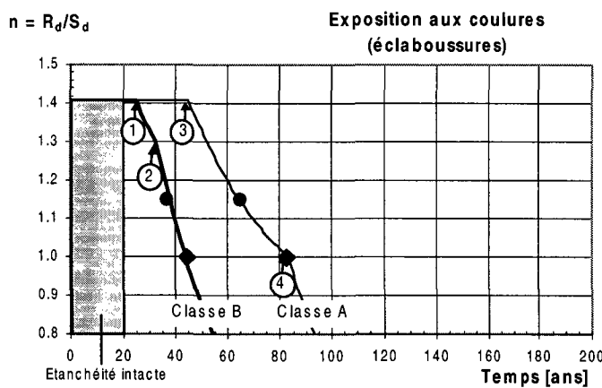
Figure 5.11 Evolution du coefficient de sécurité avec la corrosion des sections sur les béquilles en fonction de la classe de perméabilité du béton d'enrobage.
