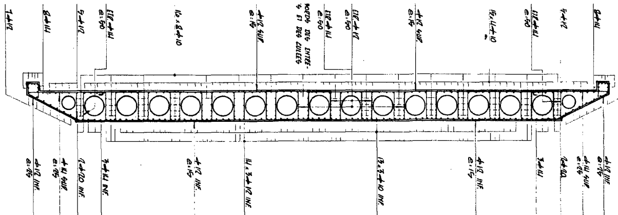
Figure 5.14 Coupes des sections sur béquille et en travée.
