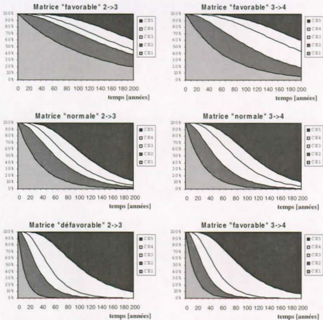
Figure 4.4 Dégradations calculées avec les matrices pour une optimisation de la transition 2 à 3 et de la transition 3 à 4.
