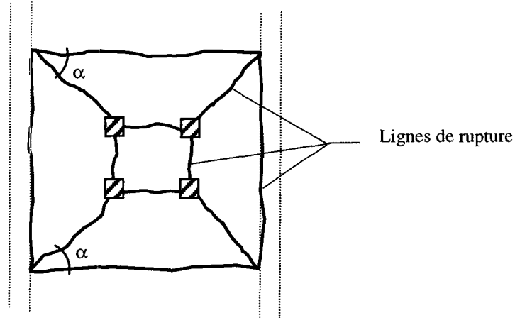
Figure 5.19 Mécanisme de rupture de la dalle du tablier en travée.
