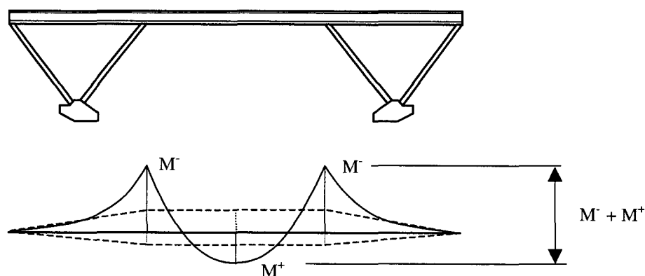
Figure 5.8 Moments dans les poutres principales
