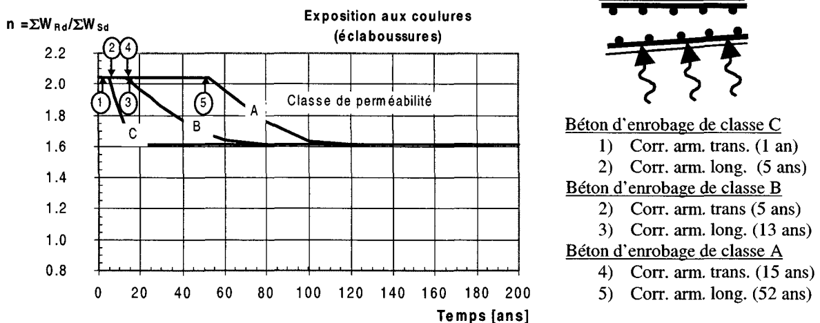
Figure 5.21 Evolution du coefficient de sécurité par la corrosion de l'armature inférieure du porte-à-faux en fonction de la classe de perméabilité du béton d'enrobage.
