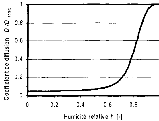
Figure 3.9 Relation entre le coefficient de diffusion et l'humidité relative ( \alpha_0 = 0.05 et h_c = 0.75 ) selon [BAZANT_71&86].
