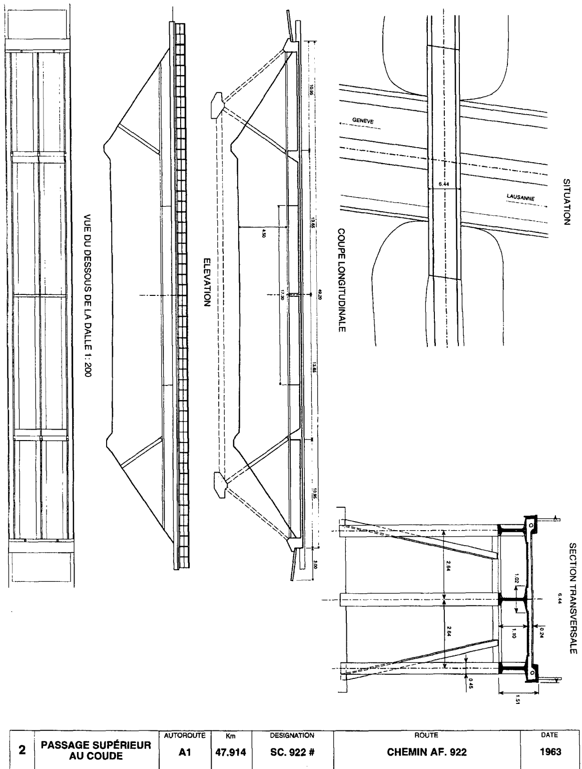
Figure A.3 Plans du pont N°2.
