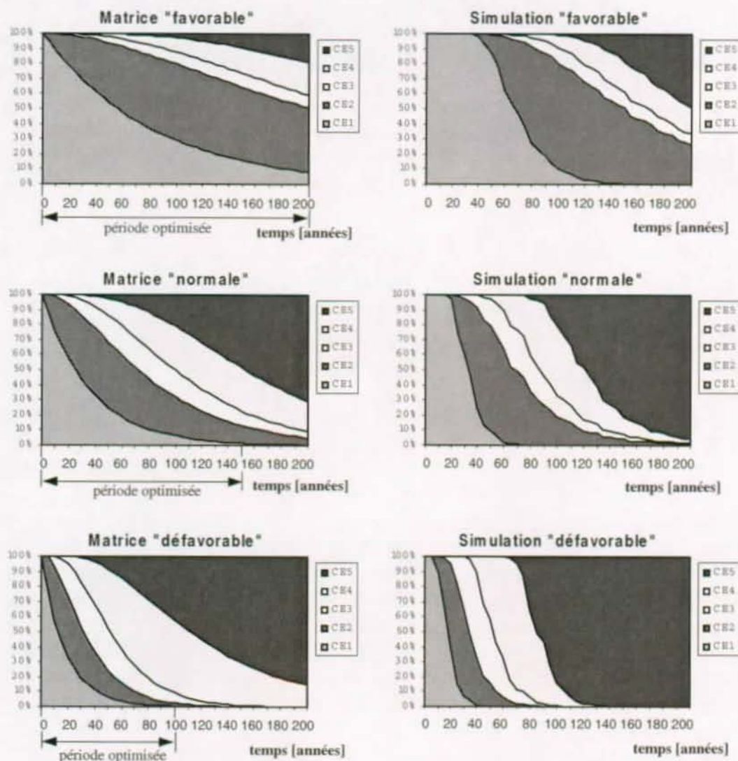
Figure 4.3 Dégradations calculées avec les matrices et les simulations numériques
