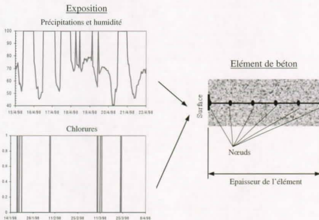
Figure 3.20 Modélisation unidirectionnelle de l'élément de béton et l'exposition de sa surface.
