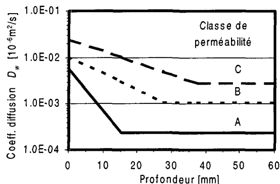
Figure 3.13 Coefficient de diffusion en fonction de la profondeur pour les trois classes de perméabilité de béton d'enrobage.
