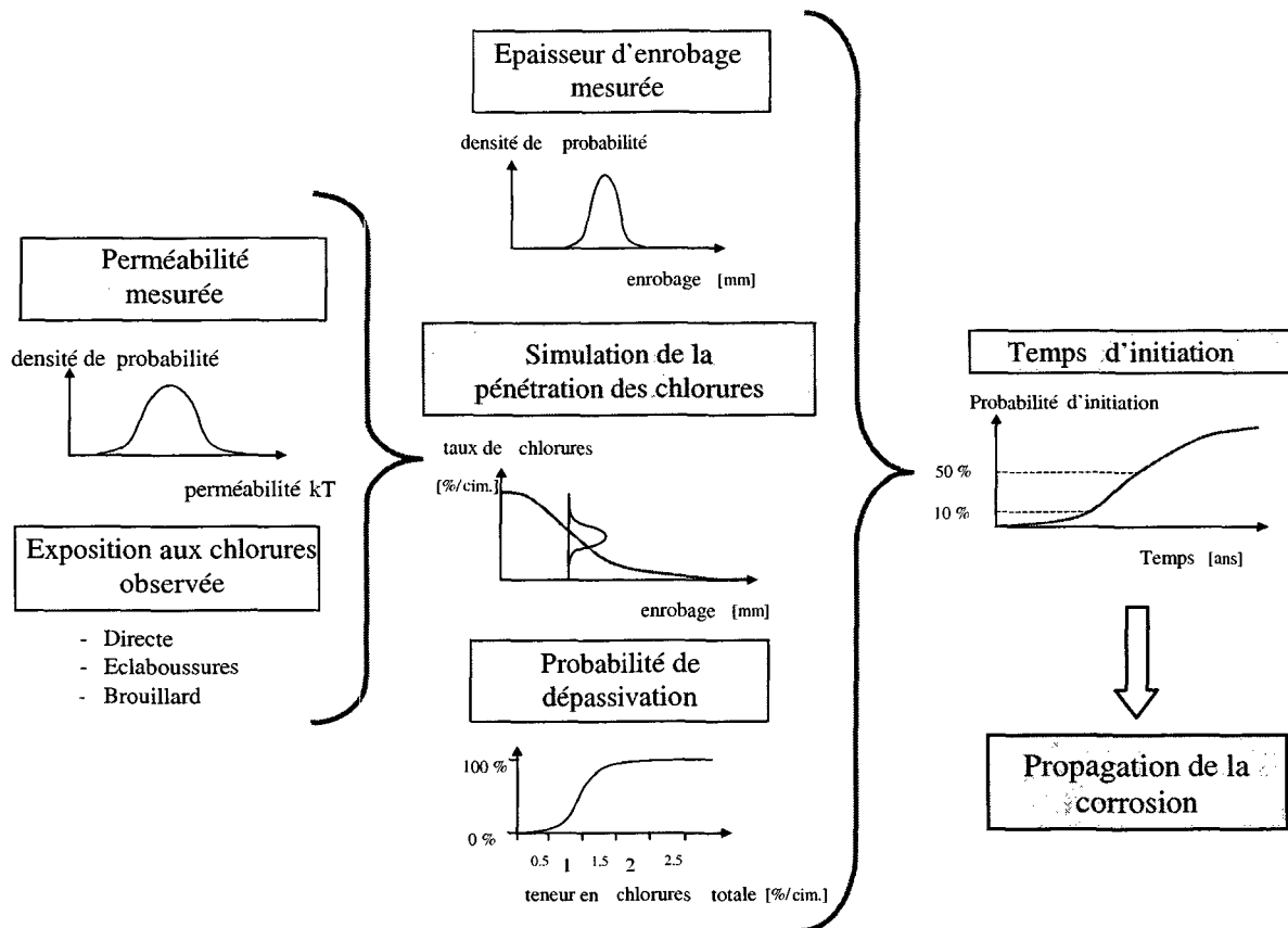
Figure 3.1 Approche probabiliste de la détérioration utilisée pour l'application du modèle développé aux ponts-routes.
