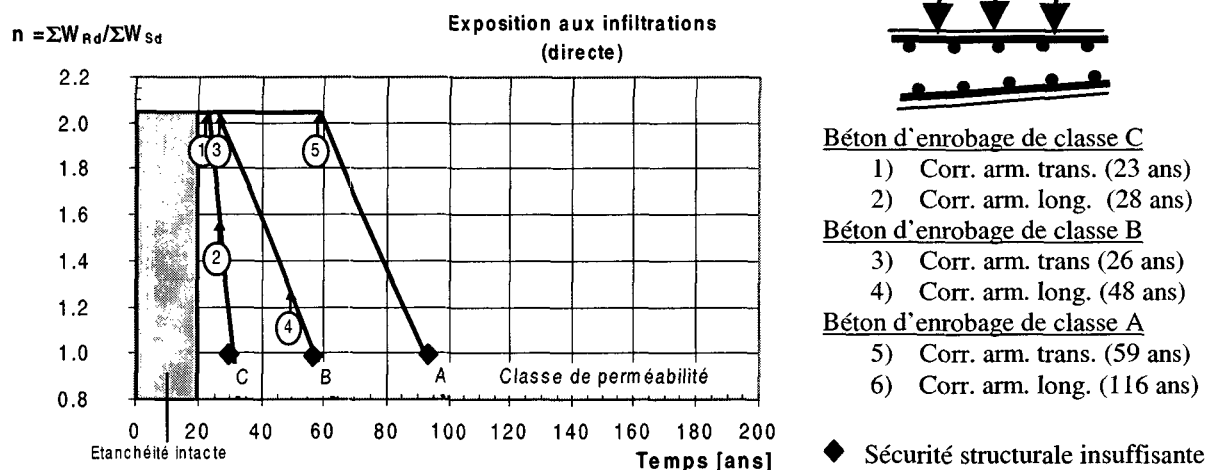
Figure 5.22 Evolution du coefficient de sécurité avec la corrosion de l'armature supérieure suite à un défaut de l'étanchéité faux en fonction de la classe de perméabilité du béton d'enrobage.
