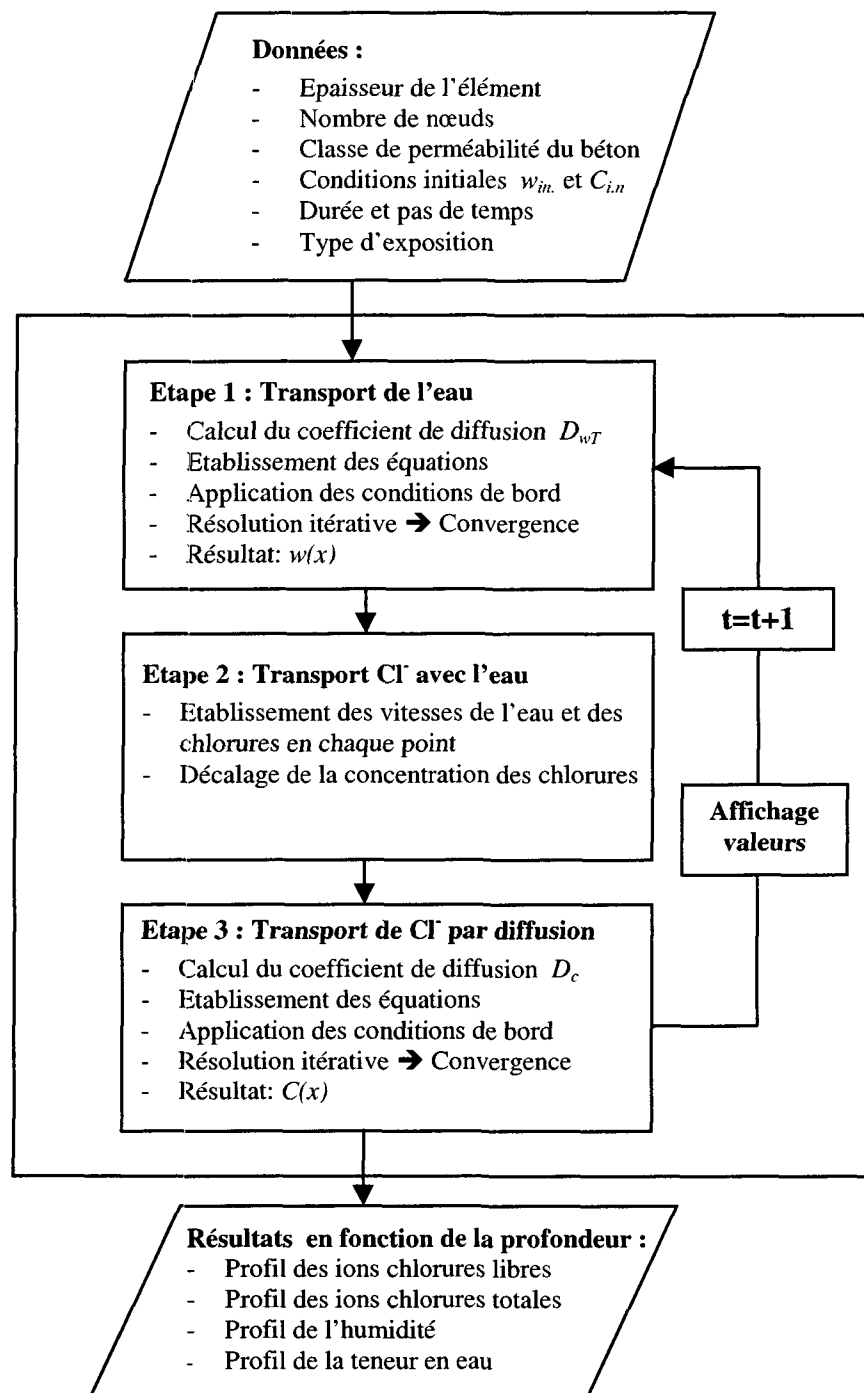
Figure 3.21 Algorithme du modèle numérique
