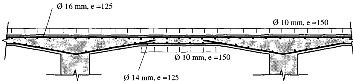
Figure 5.27 Coupe transversale du pont N°7
