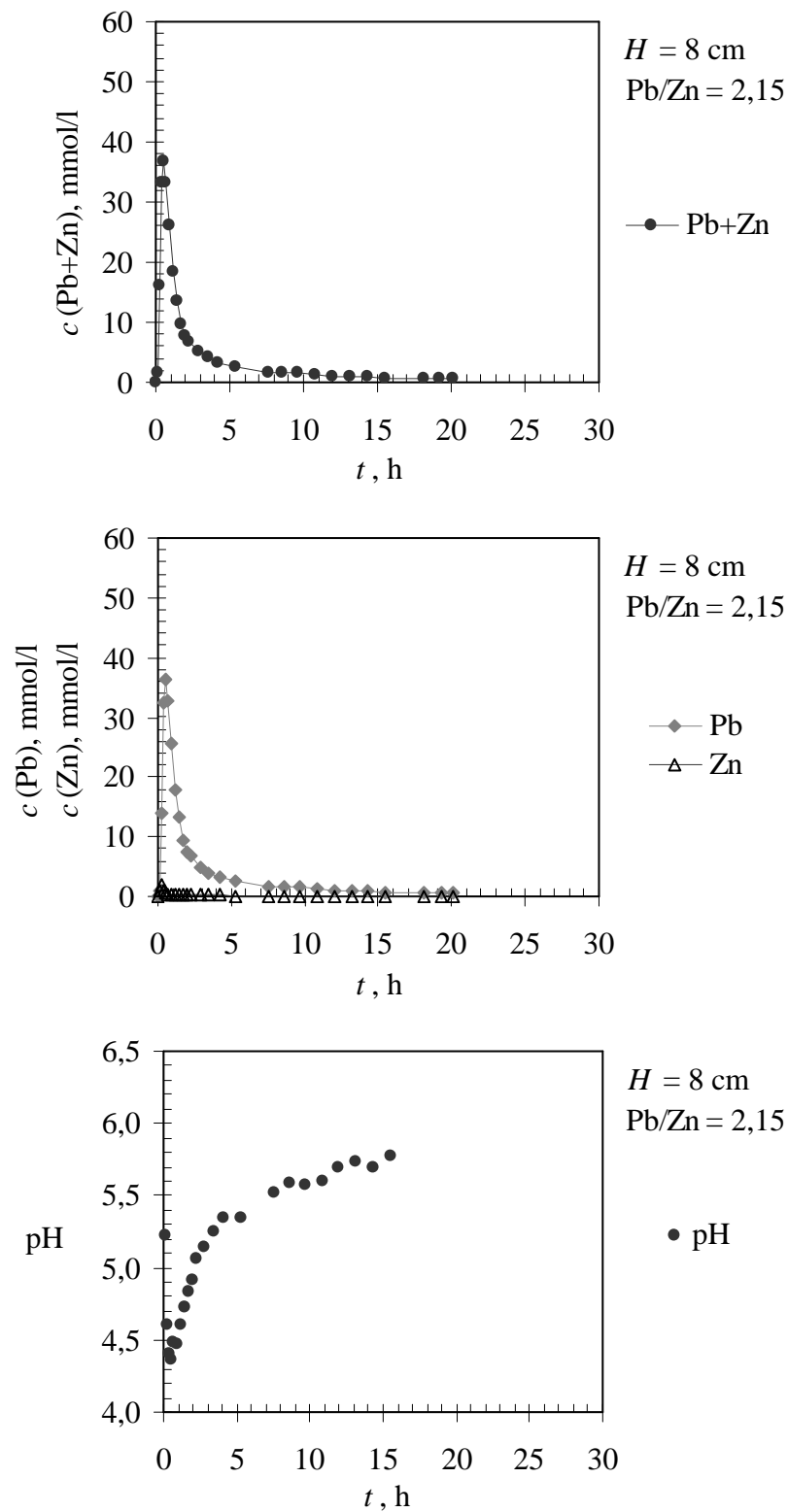
Slika 5.22. Krivulje regeneracije za visinu sloja zeolita H = 8 \text{ cm} i \text{Pb}/\text{Zn} = 2,15 za: a) ukupnu koncentraciju ( \text{Pb}+\text{Zn} ), b) pojedinačne koncentracije \text{Pb} i \text{Zn} i c) pH vrijednost.
