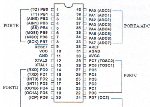
Gambar 4 Skematik Mikrokontroler ATmega8535
