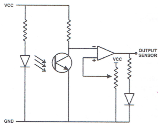
Gambar 1 Rangkaian sensor pendeteksi pelet
