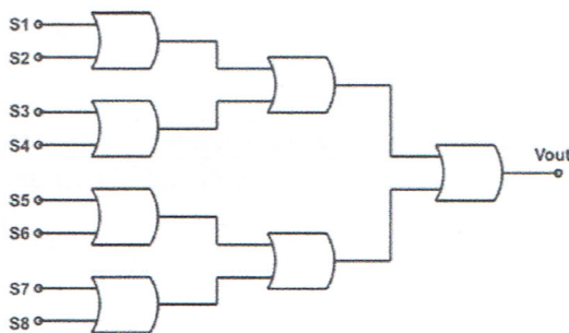
Gambar 3 Skematik penggabungan sensor
