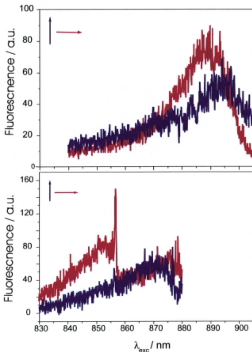
Abb. 4: Fluoreszenzanregungsspektren von LH1. Der obere Teil der Abbildung zeigt das Spektrum eines intakten Rings für zwei unterschiedliche Polarisationen des Anregungslichtes. Die leichte Verschiebung der beiden Anregungslinien deutet auf eine Aufhebung der exakten Entartung der beiden k = \pm 1 -Zustände hin, wie dies im Modell angenommen wird. Der untere Teil der Abbildung zeigt das Spektrum eines Rings, der im Verlauf der Probenpräparation zerstört wurde, so daß die Kopplung W_{nm} zwischen einigen Molekülen sehr gering wird. Dies führt zu der Beobachtung von schmalen Spektrallinien.
