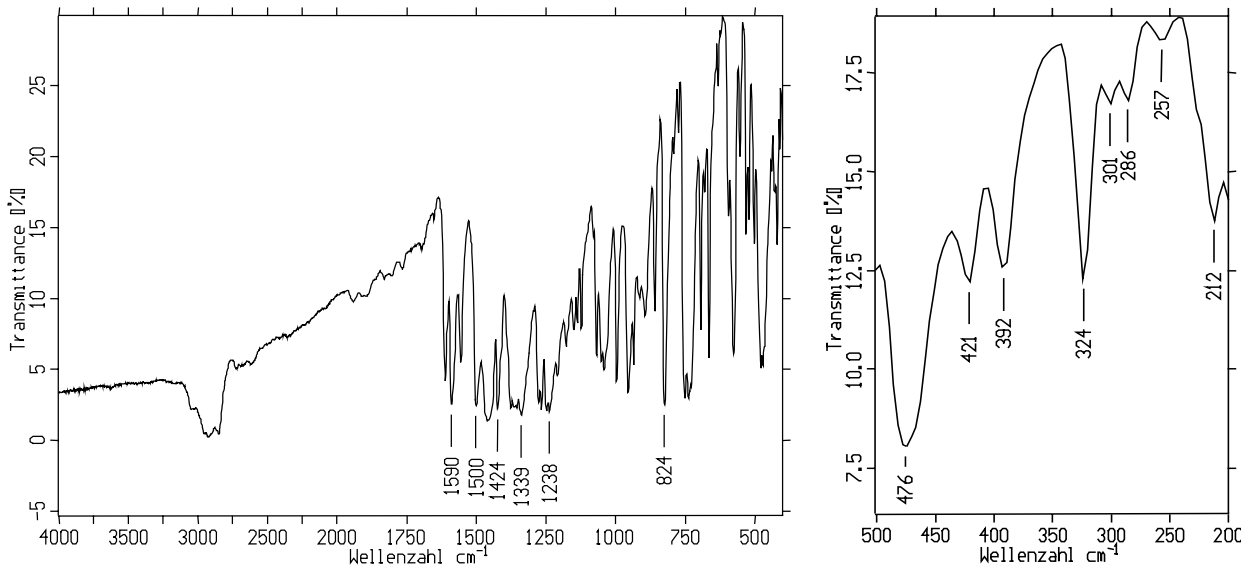
Abbildung 30: IR- und FIR-Spektrum von 11
