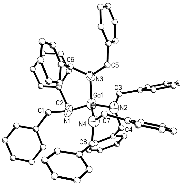
Abbildung 49: Molekülstruktur des Anions im Metallat 20 . Verbindungen 19 und 21 kristallisieren isotyp.
