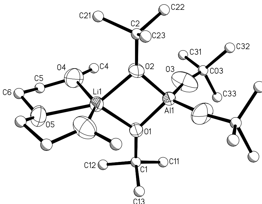
Abbildung 25: Molekülstruktur des Kontaktionenpaares in 9
