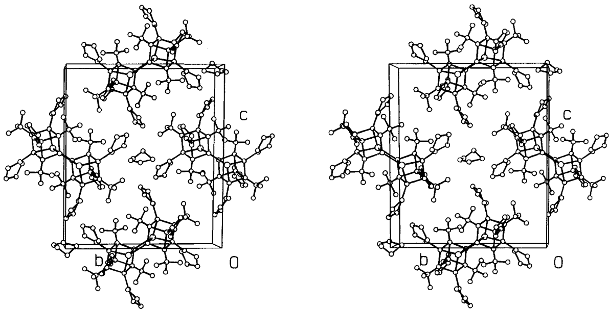
Abbildung 17: Stereoskopische Darstellung der Elementarzelle von 5
