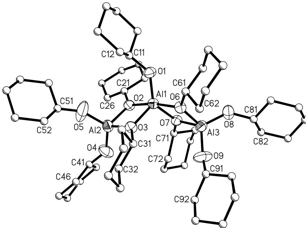
Abbildung 8: Molekülstruktur des trimeren Alkoxides 2
