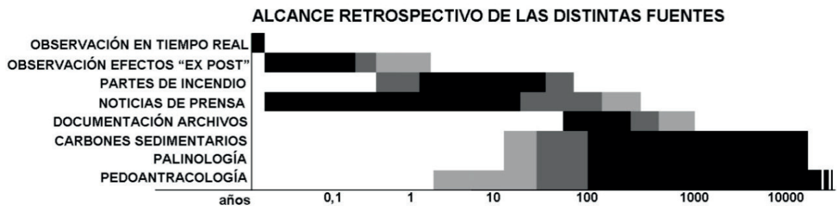
Gráfico 1. Periodo de años (antes de la actualidad) en el que las distintas fuentes resultan utilizables
