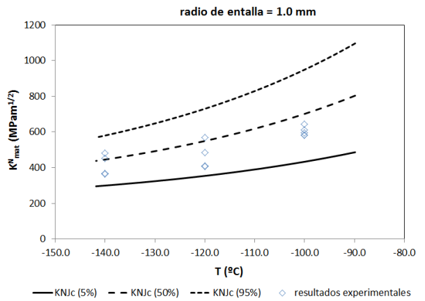
Fig. 10. Predicciones (5, 50 y 95 % de probabilidad de fallo) de la CME en probetas con \rho=1.0 mm, y comparación con resultados experimentales.
