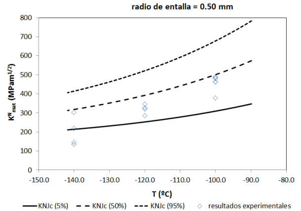
Fig. 9. Predicciones (5, 50 y 95 % de probabilidad de fallo) de la CME en probetas con \rho=0.50 mm, y comparación con resultados experimentales.
