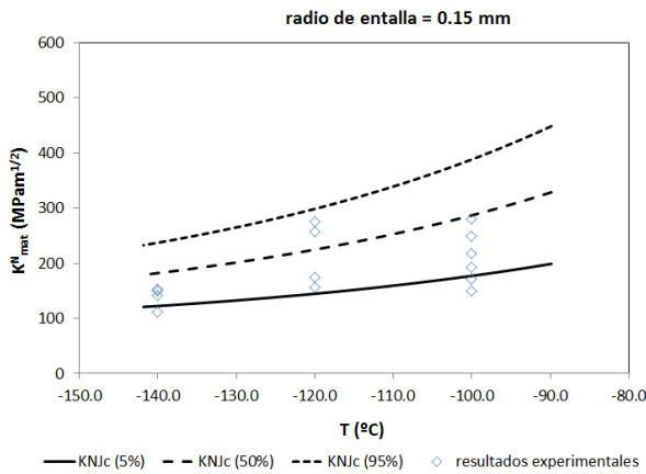
Fig. 7. Predicciones (5, 50 y 95 % de probabilidad de fallo) de la CME en probetas con \rho=0.15 mm, y comparación con resultados experimentales.
