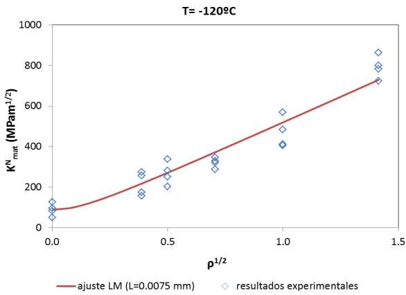
Fig. 3. Ajuste experimental según el LM de los resultados de tenacidad aparente ( L=0.0075 mm). T = -120^{\circ}\text{C} .
