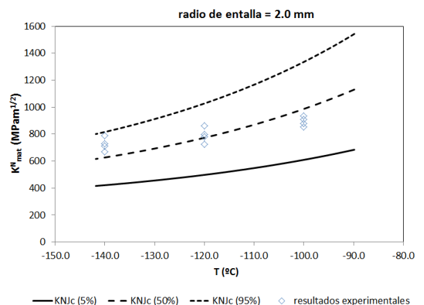
Fig. 11. Predicciones (5, 50 y 95 % de probabilidad de fallo) de la CME en probetas con \rho=2.0 mm, y comparación con resultados experimentales.
