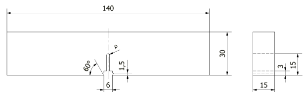
Fig.1. Geometría de las probetas SENB entalladas. \rho varía entre 0 mm y 2.0 mm.
