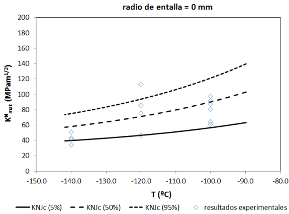
Fig. 6. Predicciones (del 5, 50 y 95 % de probabilidad de fallo) de la CME en probetas con \rho=0 mm, y comparación con resultados experimentales.
