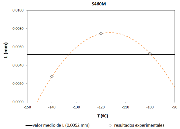
Fig. 5. Valores de L obtenidos del ajuste experimental, valor medio de L considerado en los cálculos (0.0052 mm), y ajuste polinómico de L .
