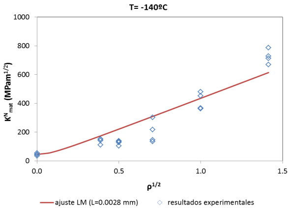
Fig. 4. Ajuste experimental según el LM de los resultados de tenacidad aparente ( L=0.0028 mm). T = -140^{\circ}\text{C} .
