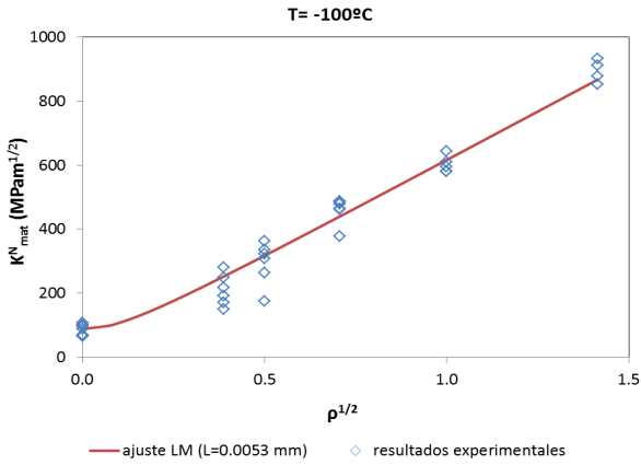
Fig. 2. Ajuste experimental según el LM de los resultados de tenacidad aparente ( L=0.0053 mm). T = -100^{\circ}\text{C} .
