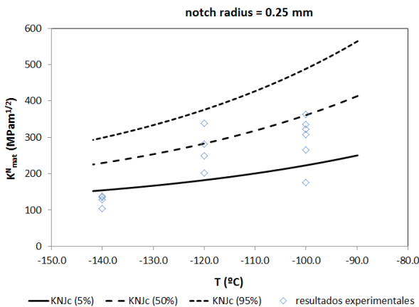
Fig. 8. Predicciones (5, 50 y 95 % de probabilidad de fallo) de la CME en probetas con \rho=0.25 mm, y comparación con resultados experimentales.
