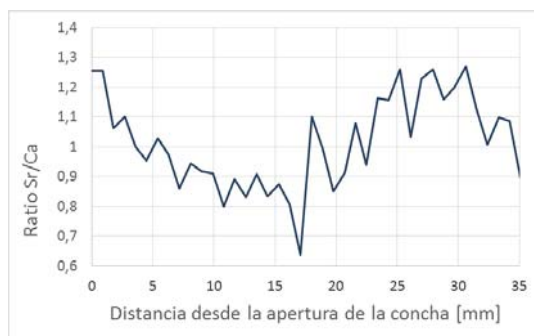
Fig. 4: Secuencias de los ratios Mg/Ca y Sr/Ca en dos ejemplares diferentes de Phorcus lineatus .
