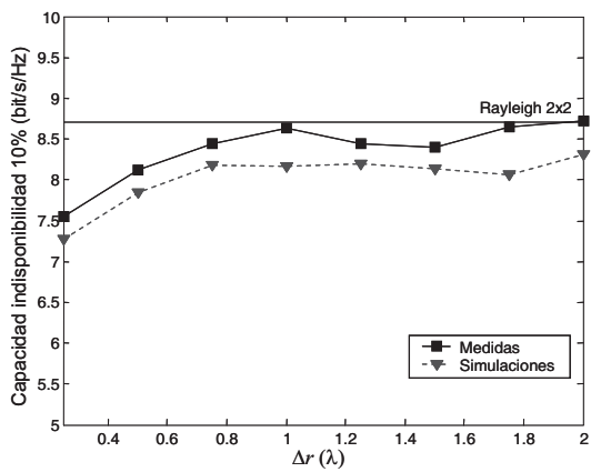
Fig. 5. Capacidad de indisponibilidad en escenario abierto (LOS, arrays paralelos).
