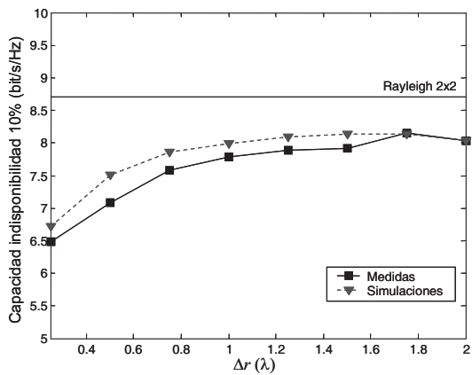
Fig. 6. Capacidad de indisponibilidad en escenario de oficinas (LOS, arrays paralelos).
