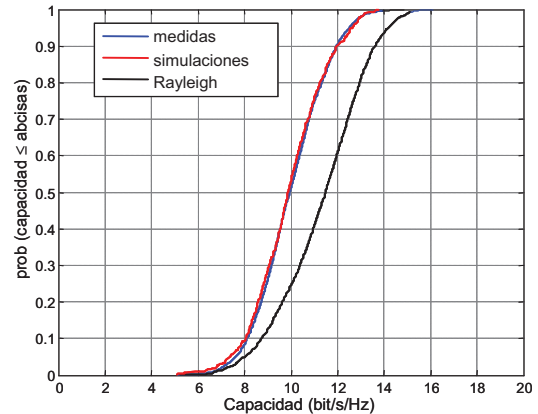
Fig. 1. Capacidad en escenario abierto (LOS, arrays perpendiculares, \Delta r = \lambda , SNR=20 dB).
