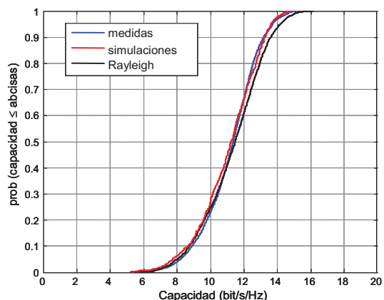
Fig. 3. Capacidad en escenario abierto (NLOS, arrays perpendiculares, \Delta r = \lambda , SNR=20dB).
