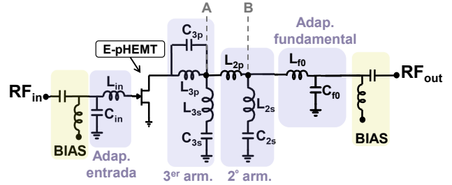
Fig. 2. Esquemático simplificado del amplificador clase E.
