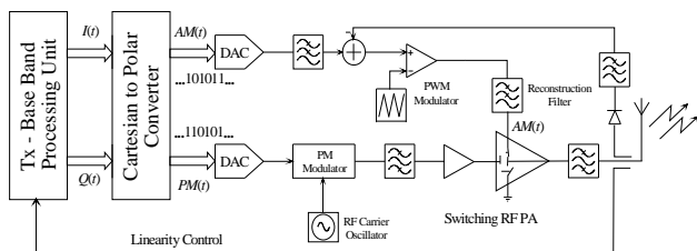
Fig. 3. Esquema simplificado de un Tx polar.
