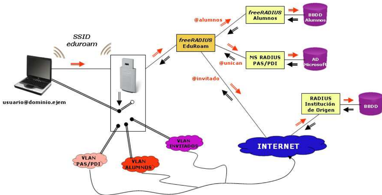
Fig. 2. Esquema general del desarrollo de red inalámbrica adoptado en la Universidad de Cantabria
