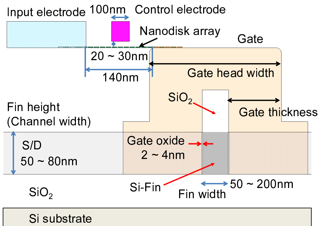
図 3.4 NDA-FinFET 断面模式図.
