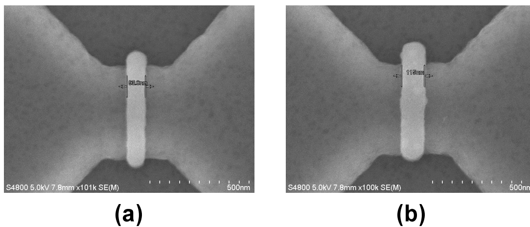
図 3.10 EB 露光後ゲートパターンの SEM 観測結果 : (a) 設計値 50nm, (b) 設計値 80nm.
