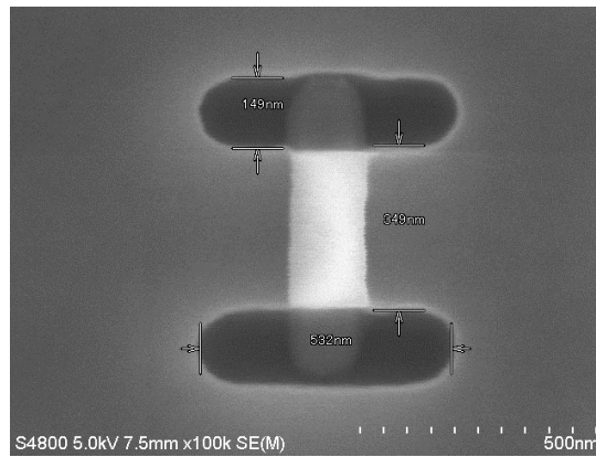
図 3.21 NDA-AI コンタクトホールの SEM 観測結果.
