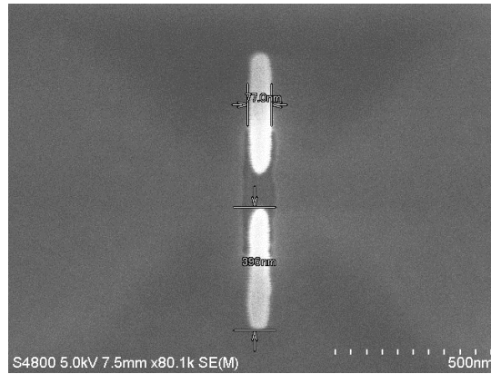
図 3.19 NDA ドライエッチング後 SEM 観測結果.
