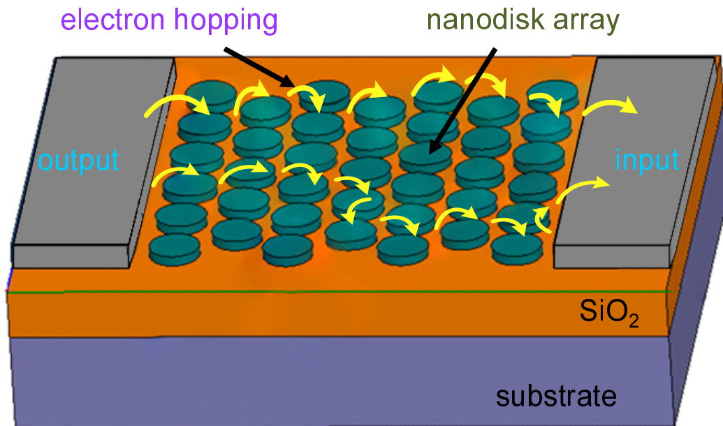
図 3.1 NDA 構造.
